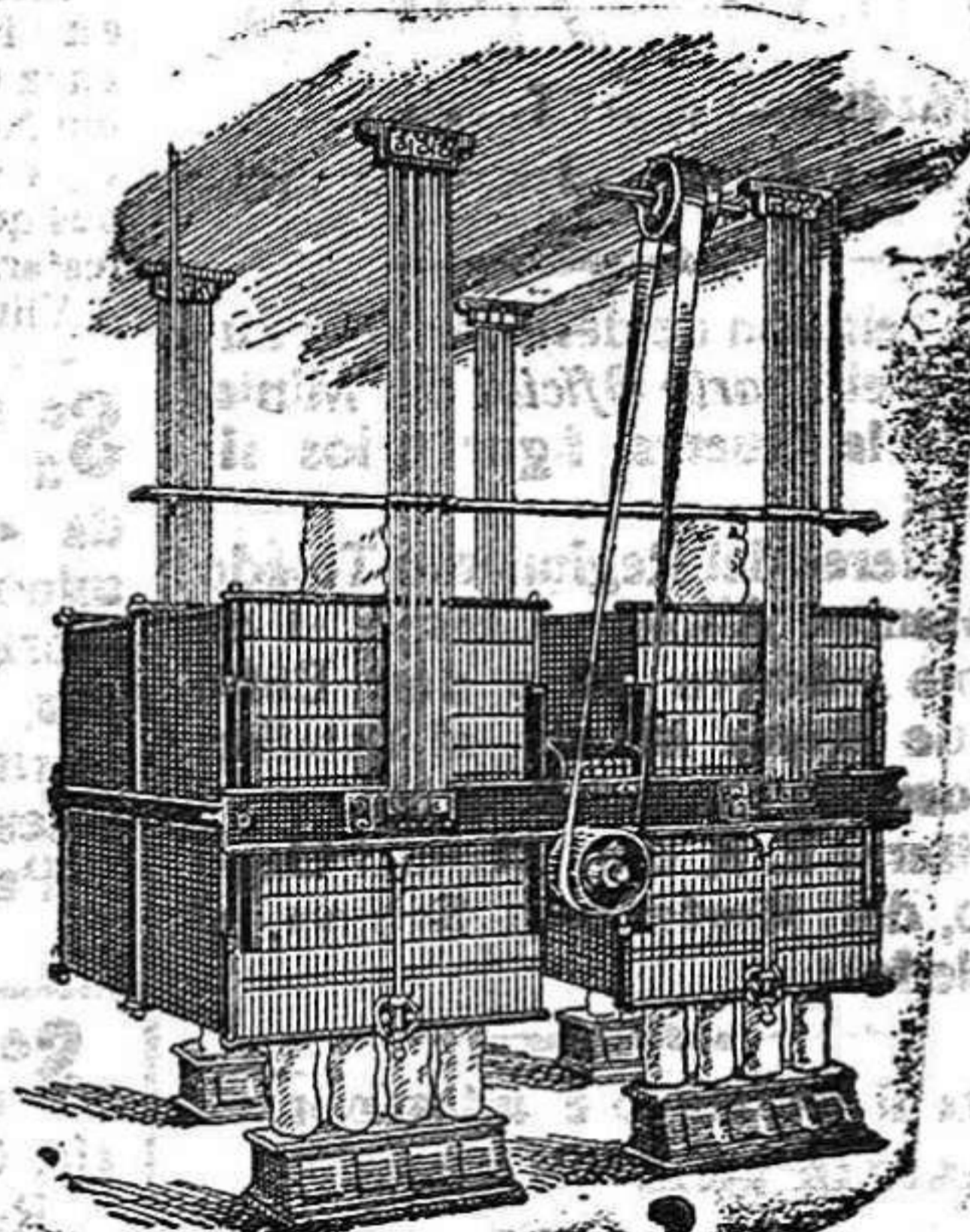
Nuevo planchete de libre oscilación y equilibrio automático.—Privilegio Buhler.
