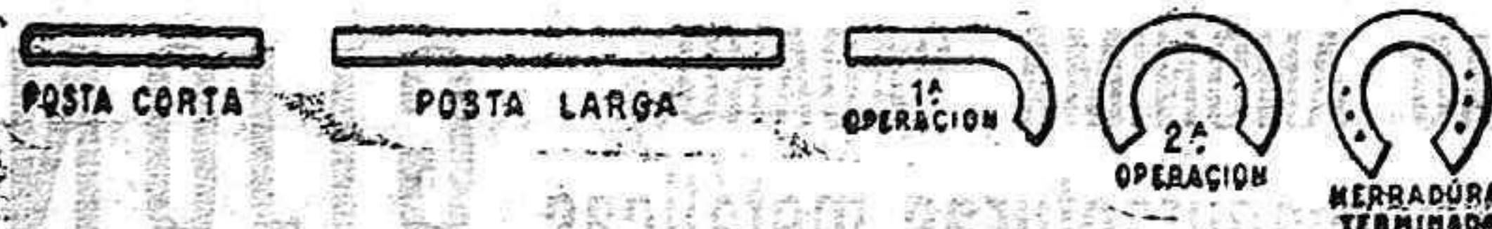
RECORTES Y PLETINAS PARA FABRICACIÓN DE HERRADURAS.
