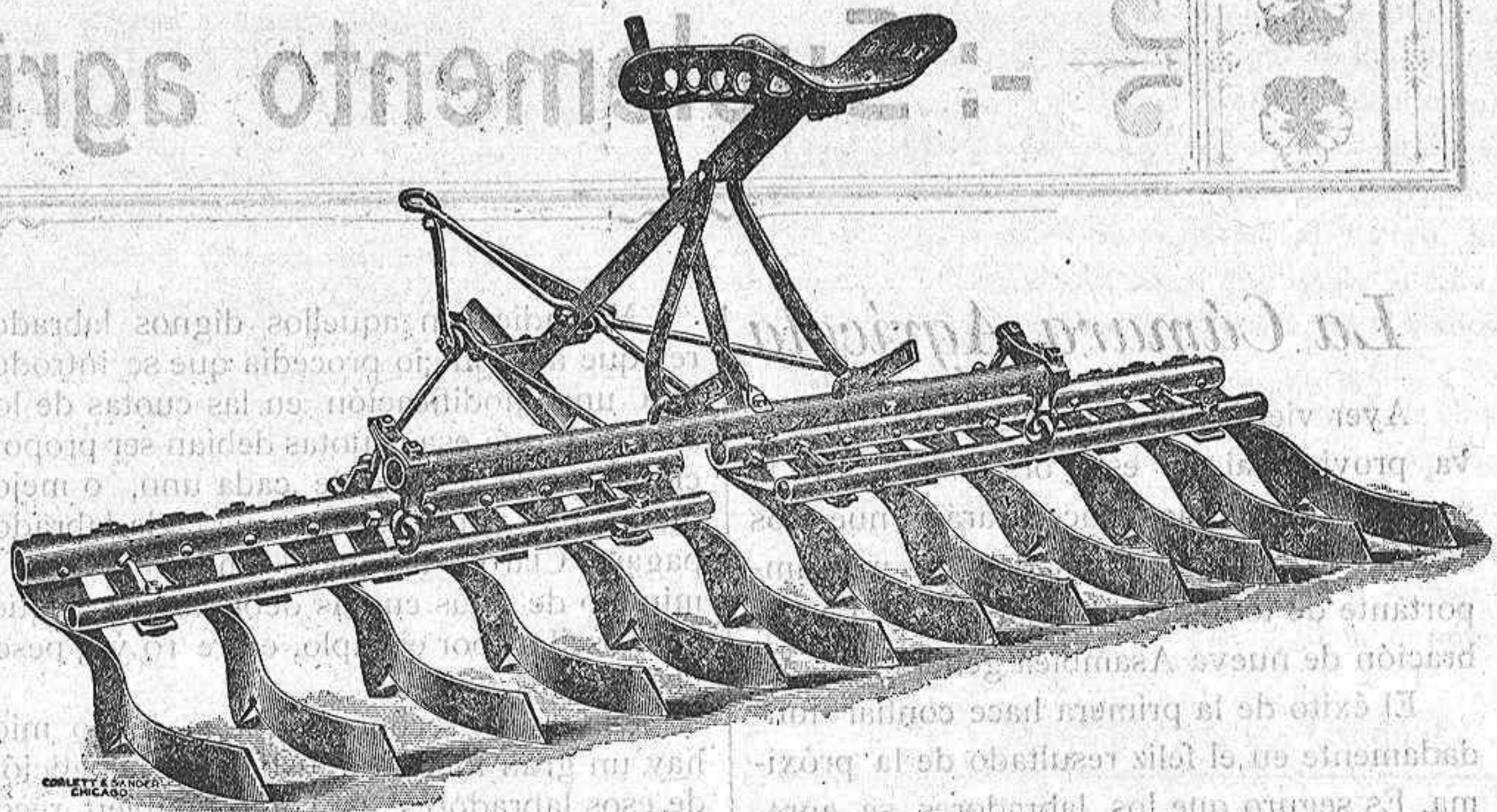
GRADA «ACME» DE DOCE CUCHILLAS
