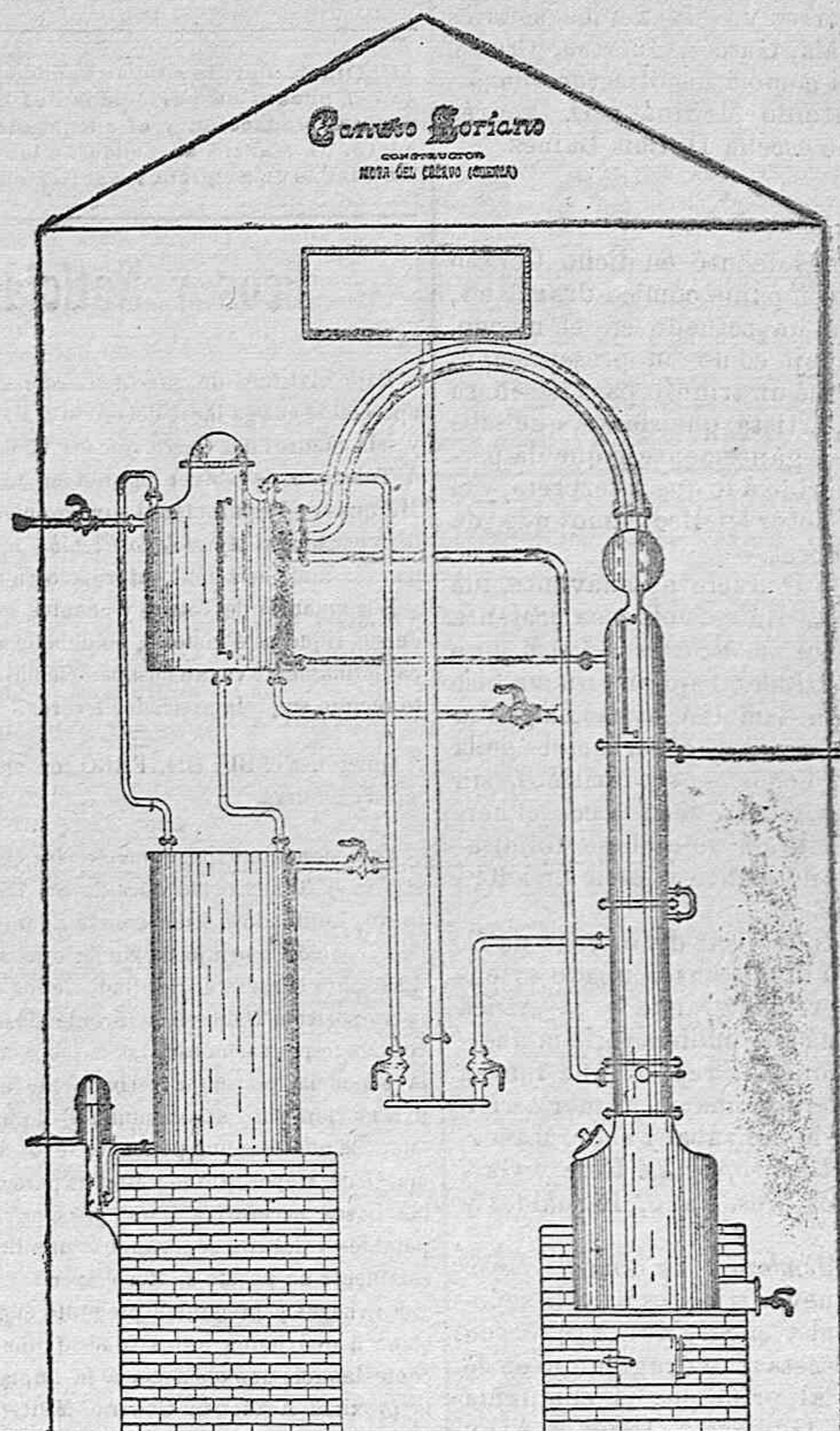
Aparato SISTEMA GIESVER para la quema de orujos, madres, vinos picados, produciendo alcoholes en su rectificación de 95 á 96 grados. Precio del mismo, de 650 litros de cubida 2.750 pesetas, montado y garantizada su buena marcha y la buena clase de alcohol de su producción.
