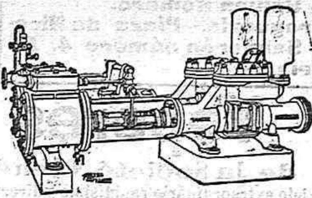
Bomba "Tangyes".
