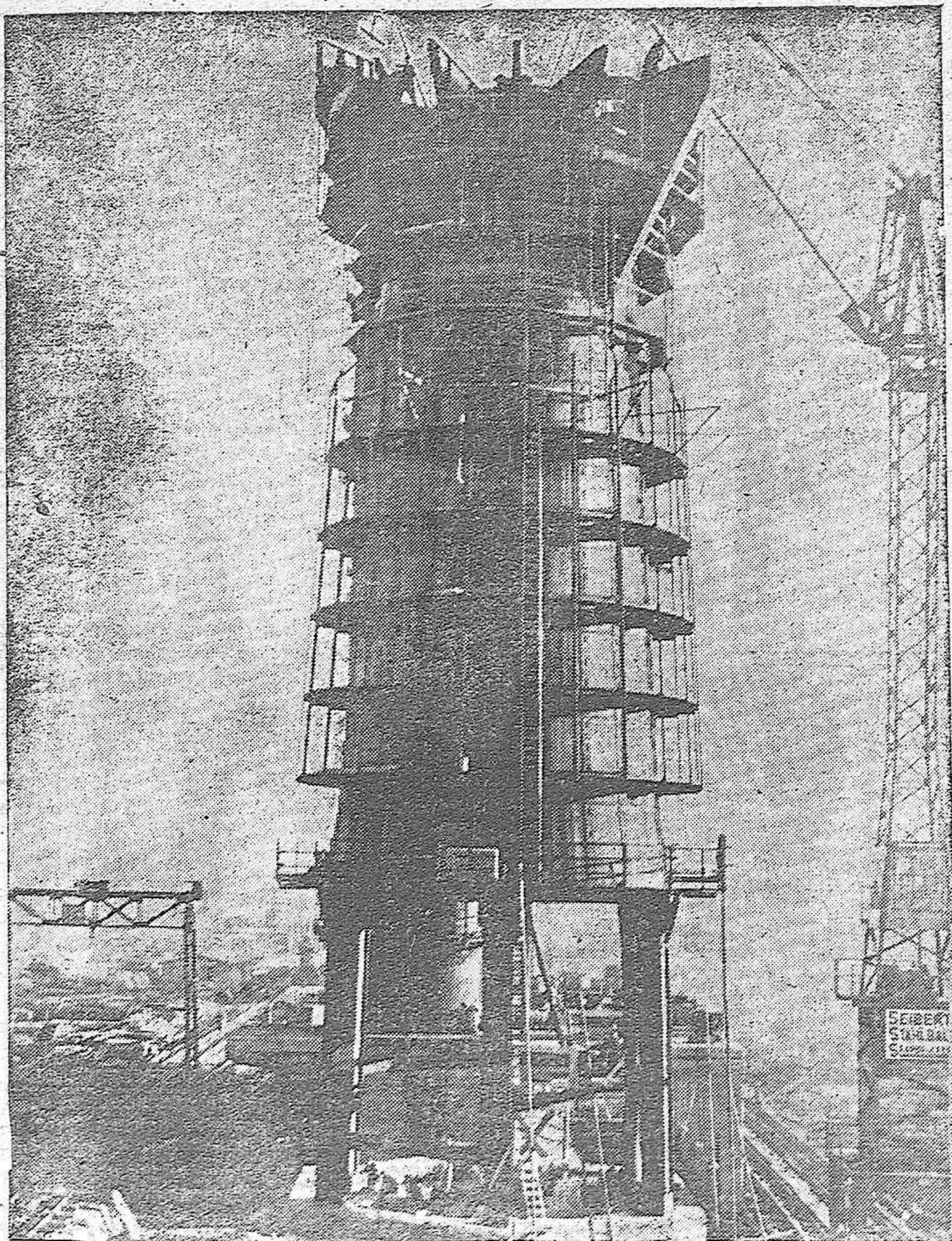
LOS GRANDES ESTABLECIMIENTOS SIDERURGICOS DEL REICH «HERMANN GORING». — En ejecución del programa del Plan Cuádruple, se encuentran en explotación los yacimientos de hierro de las montañas del Harz. La foto nos presenta un Alto Horno en construcción
