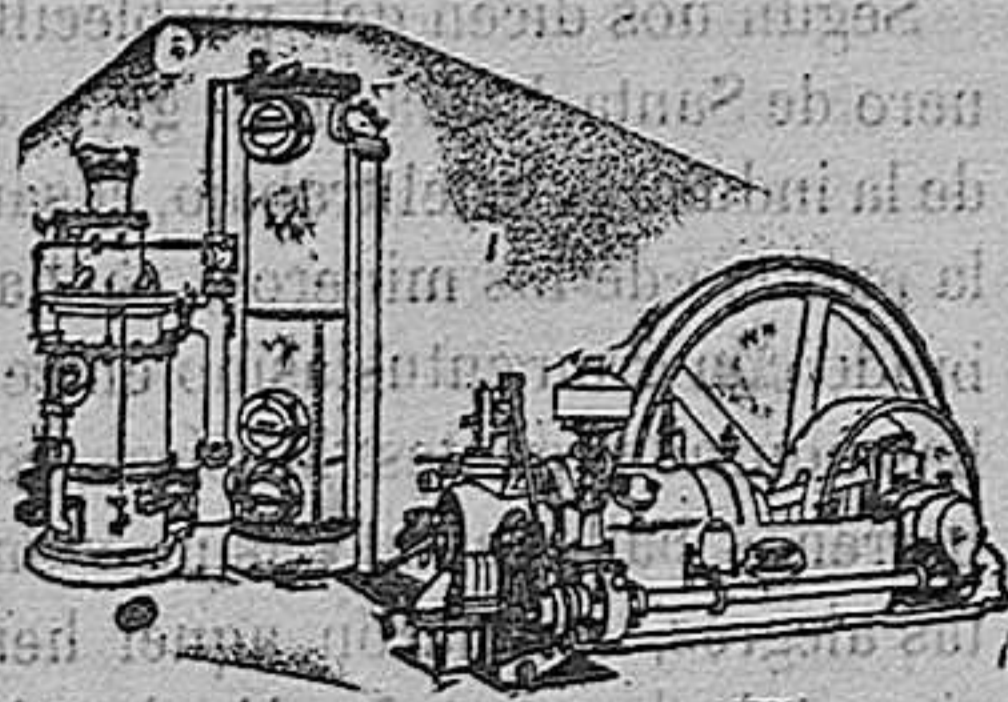
Motor de Gas Pobre por Aspiración "Tangyes"
