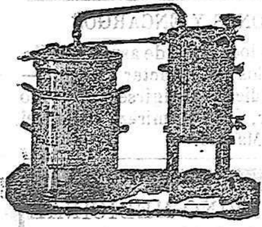
Alambique.
