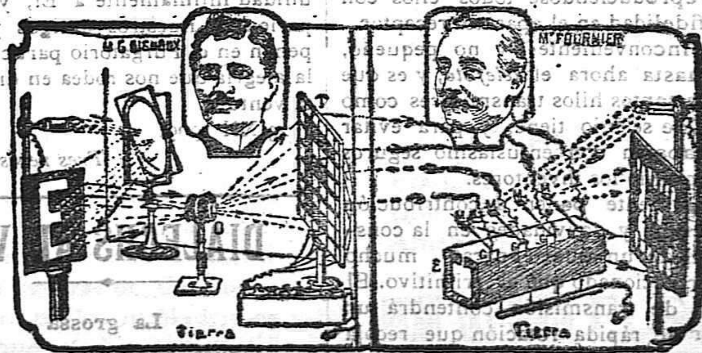
DISPOSICIÓN DEL TELEFOTO: O. Objetivo.—T. Cuadro de células de Selenio.—M. M. Espejos.—G. Galvanómetro.—C. Electroímán.
