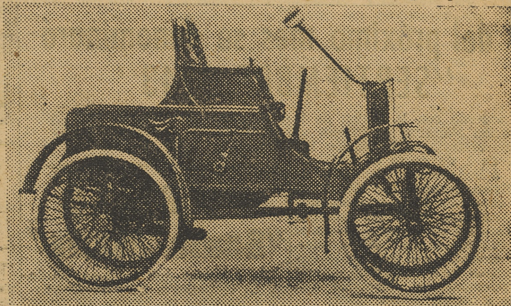
Un coche construido en Warren, Ohio (Estados Unidos), en noviembre 6 de 1899. Posee un motor de un cilindro con transmisión a correa, con tres velocidades
