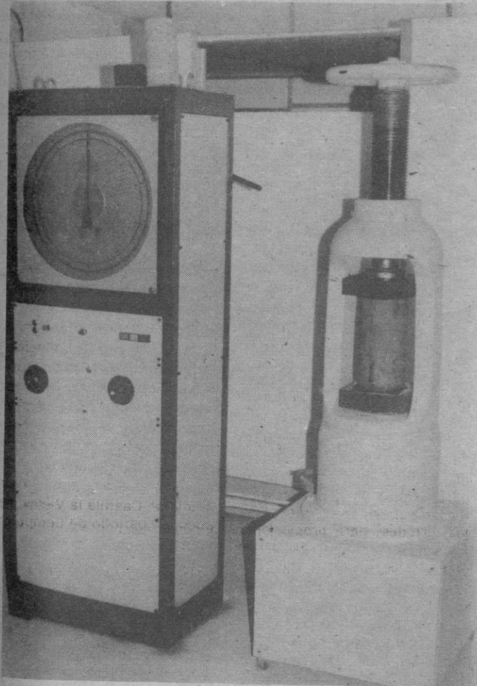
Con esta prensa se mide la resistencia del hormigón, previamente humidificado.
