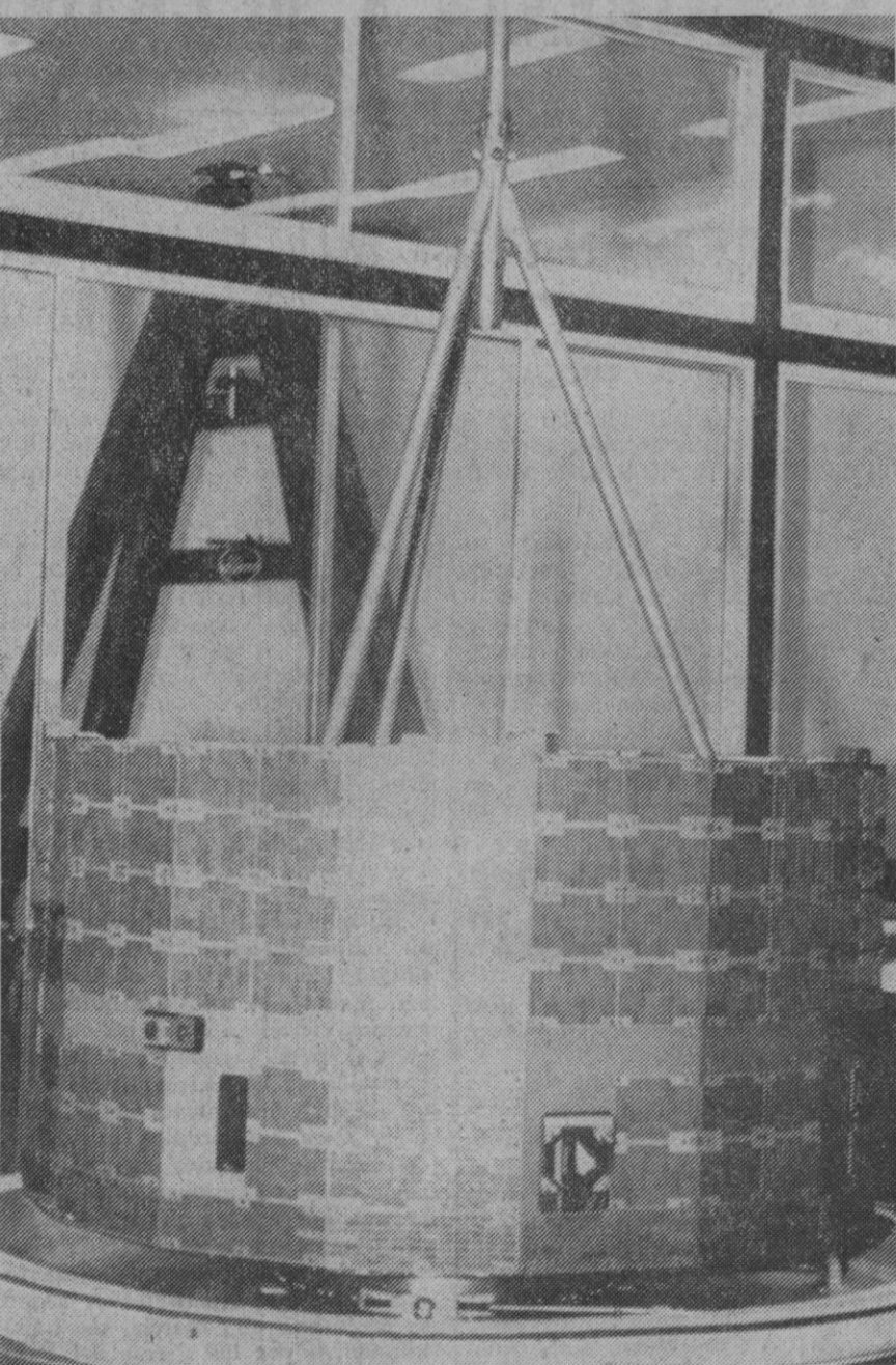
Madrid.—Estructura del satélite «Heos A-2» en la factoría de Getafe de C. A. S. A. antes de su envío a M. B. B. de Alemania. Este satélite se encuentra ya orbitando la Tierra. Tiene por objeto el estudio del campo magnético terrestre y de la distribución de partículas energéticas en el espacio. En el proyecto han cooperado la empresa Messerschmitt-Bolkow-Blohm y Construcciones Aeronáuticas, S. A.—(Telefoto Europa Press)
