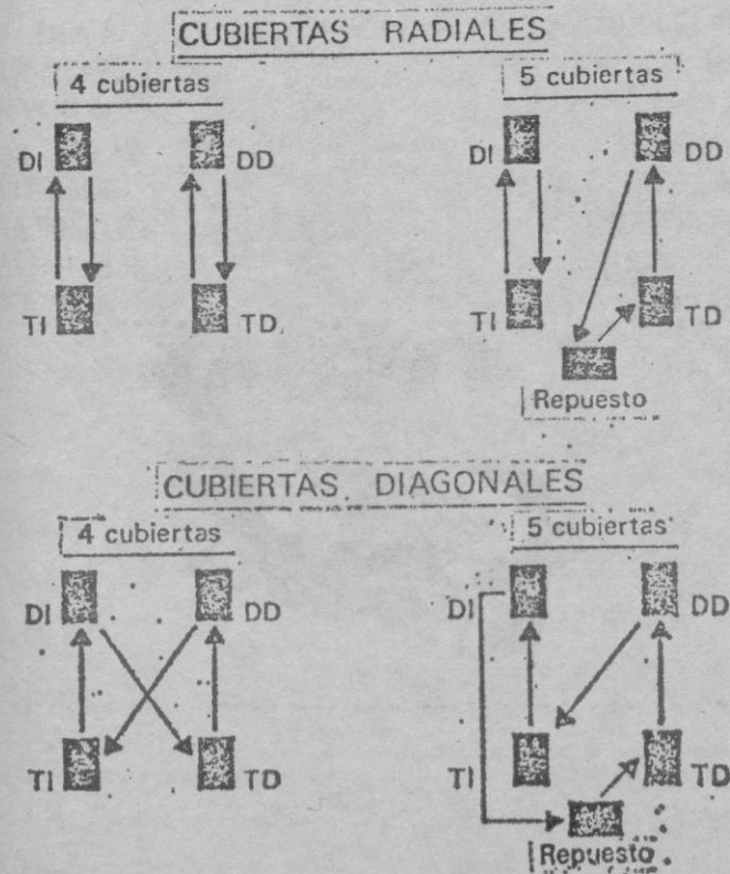
EN EL GRABADO, LA EXPLICACION IDEAL PARA AUMENTAR LA VIDA DE UNOS NEUMATICOS. EN EL GRABADO SUPERIOR, CUBIERTAS RADIALES; EN EL INFERIOR, DIAGONALES.
