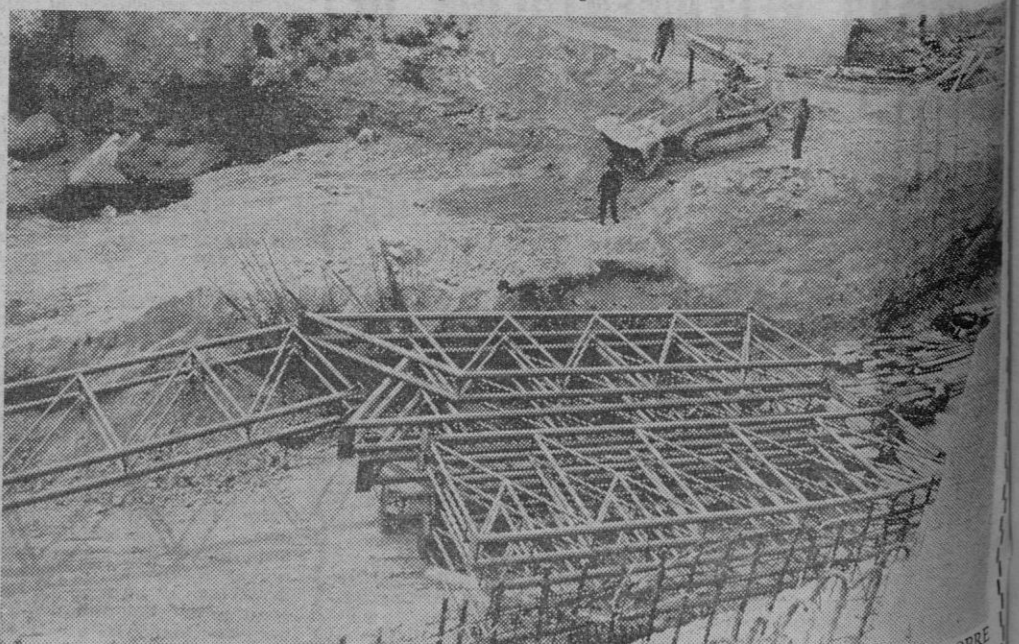
PRIMERA REMESA DEL MATERIAL QUE HA DE FORMAR EL PUENTE PROVISIONAL SOBRE LA PLAZA MAYOR. LLEGO AYER A SU DESTINO. LA SUSPIRADA SOLUCION DE EMERGENCIA ES COSA DE DIAS — (FOTO JUANET)
