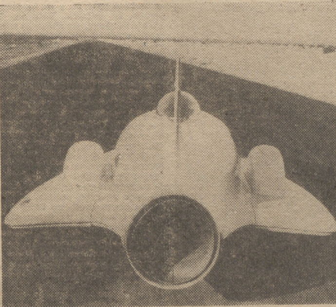
Visto desde la cola, este turborreactor americano semeja mucho más a un avión-cohete que a un automóvil. (Foto Cifra.)
