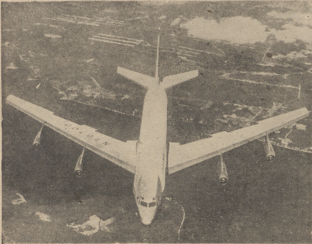
El transporte de propulsión a chorro Boeing, retratado durante su primer vuelo desde Renton Wash., y que permaneció en el aire una hora y veinticuatro minutos. Tiene una velocidad de crucero de 550 millas por hora, envergadura, 130 pies, y longitud de 128 pies. Hará el viaje Londres-Nueva York en menos de siete horas, con capacidad para 80 a 130 pasajeros y altitud operacional de 30.000 a 40.000 pies. (Foto Torrecocha.)
