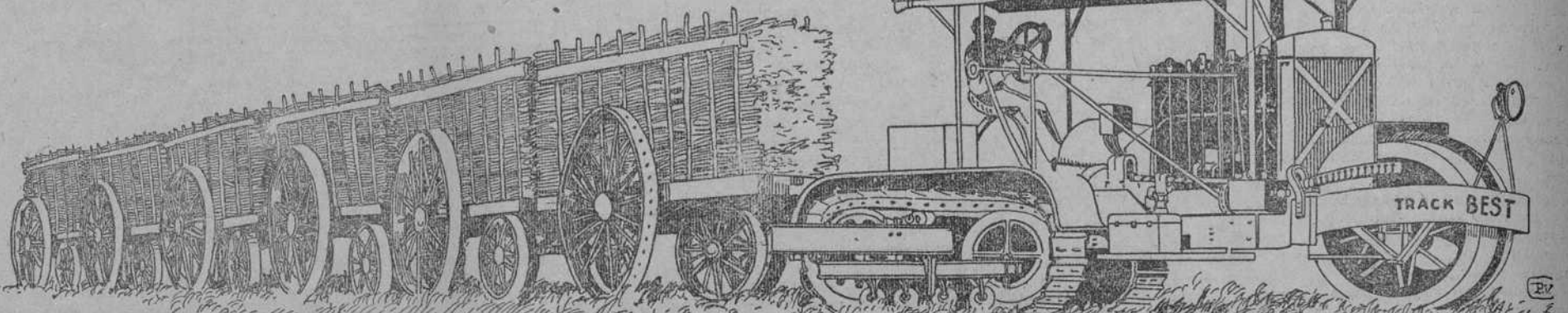
Tractor "TRACKLAYER", de 75 HP., tirando 6 carros de caña, en la finca Santa Ana, del señor Juan Mila, de Sagua la Grande
