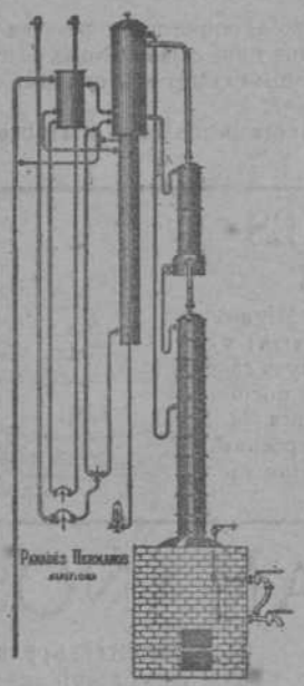
Aparato destilación continua á fuerza directa. Producción del alcohol de 95 á 96°, ó sean 40° Cartier.
