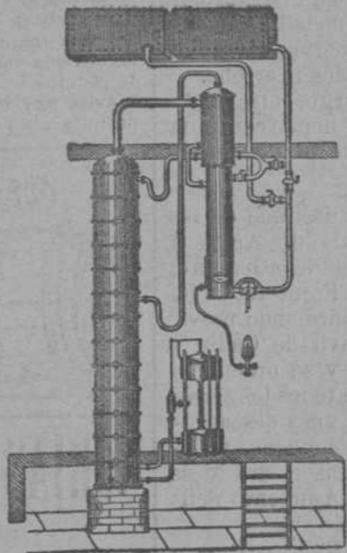
Aparato de destilación continua á vapor. Producción del alcohol de 95 á 96°, ó sean 40° Cartier.
