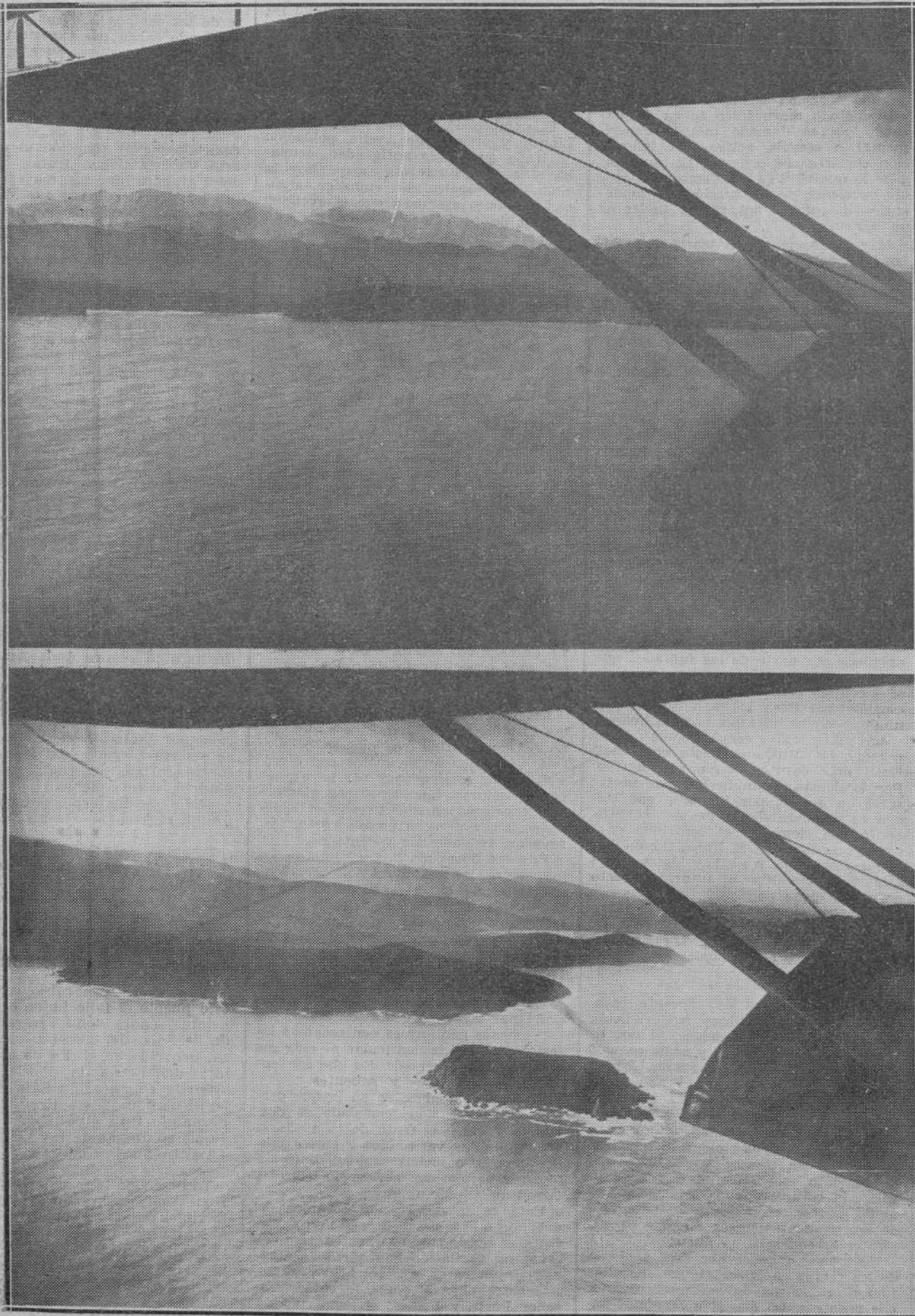
Detalle de la costa frente a San Vicente de la Barquera.—Al fondo, los macizos de los Picos de Europa.—En la parte inferior un detalle de la costa asturiana.
