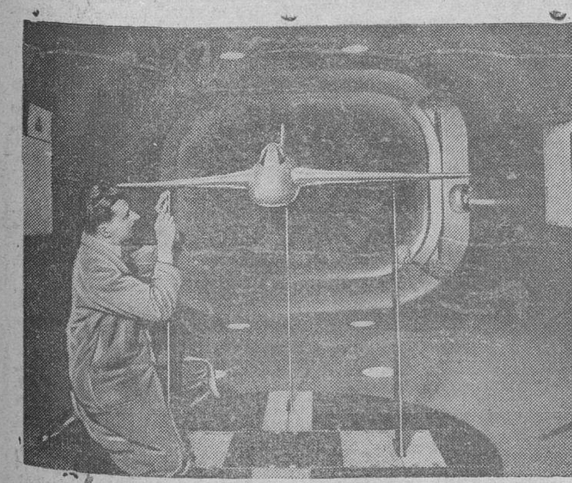
Montaje de un modelo en posición dentro del túnel aerodinámico. En esta prueba, se somete el modelo a una corriente de aire a una velocidad de 960 kilómetros por hora. (Foto Calpe).
