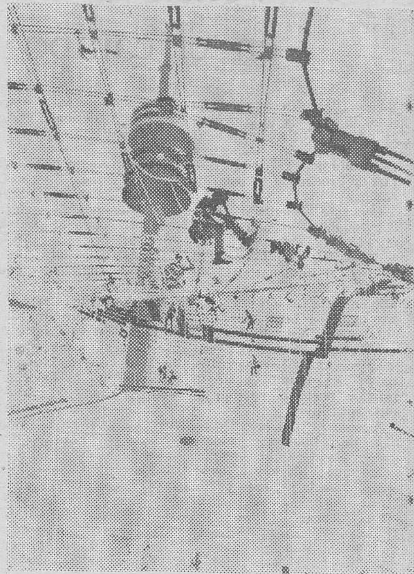
Un año antes de los Juegos Olímpicos: el techo olímpico sobre el estadio, el Palacio de los Deportes y el estadio de natación será cubierto. Debajo de la red del tejado cuelga una capa aisladora de lámina transparente. Luego será atornillada la red de cables con placas de vidrio acrílico.
