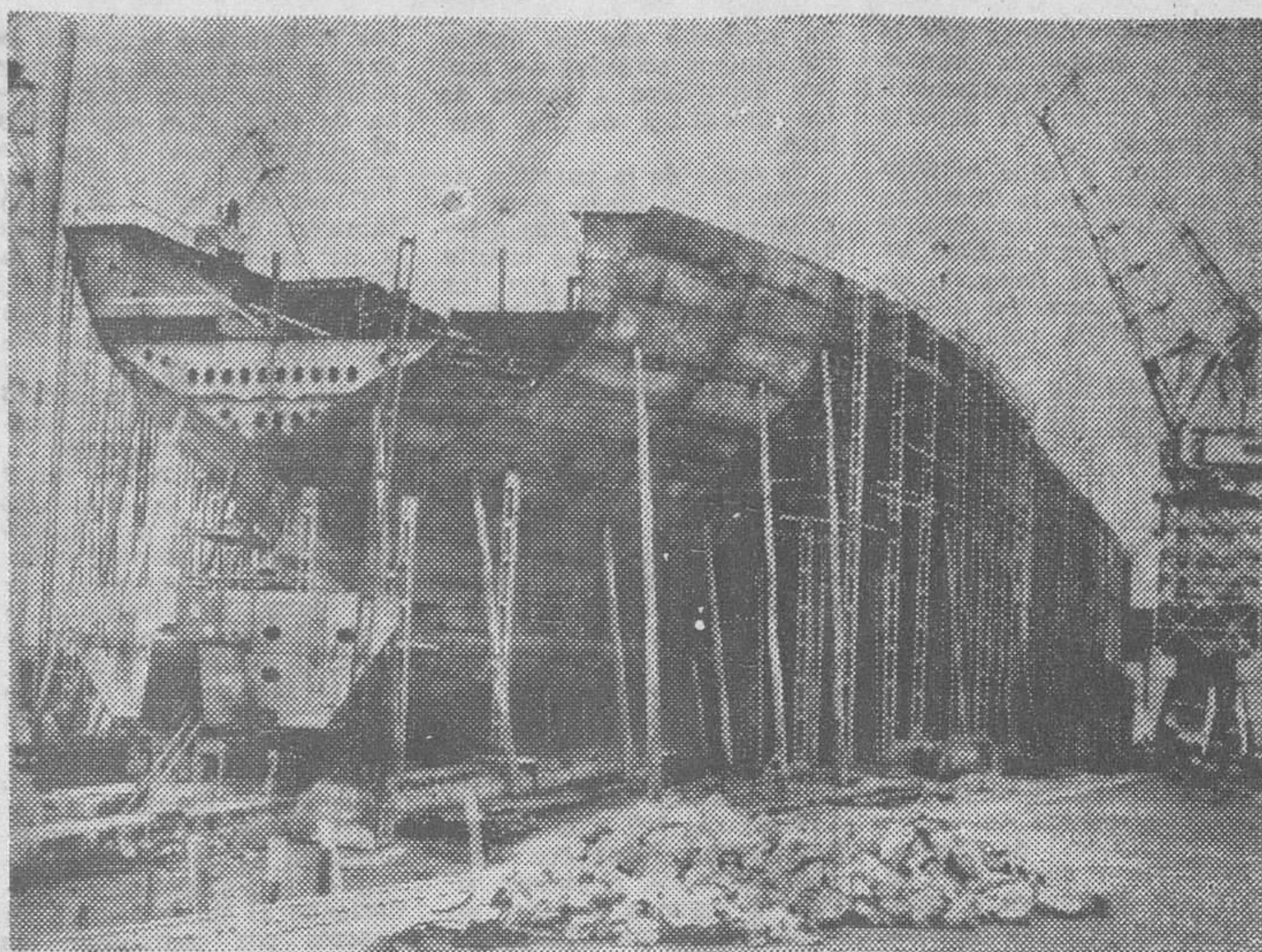
En los astilleros Astano de La Coruña se está construyendo el mayor petrolero de España, el «Centas», de 91.000 toneladas. Dicho buque irá equipado con un sistema complejo de mando auto-eléctrico, dotado con su brújula giroscópica. En la foto, vista del futuro petrolero en plena construcción (Foto CIFRA)
