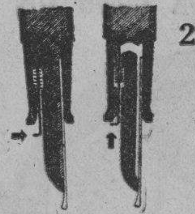
2. Cierre hermetico de la tinta. Evita la gotera y el chorro en la tapa.
