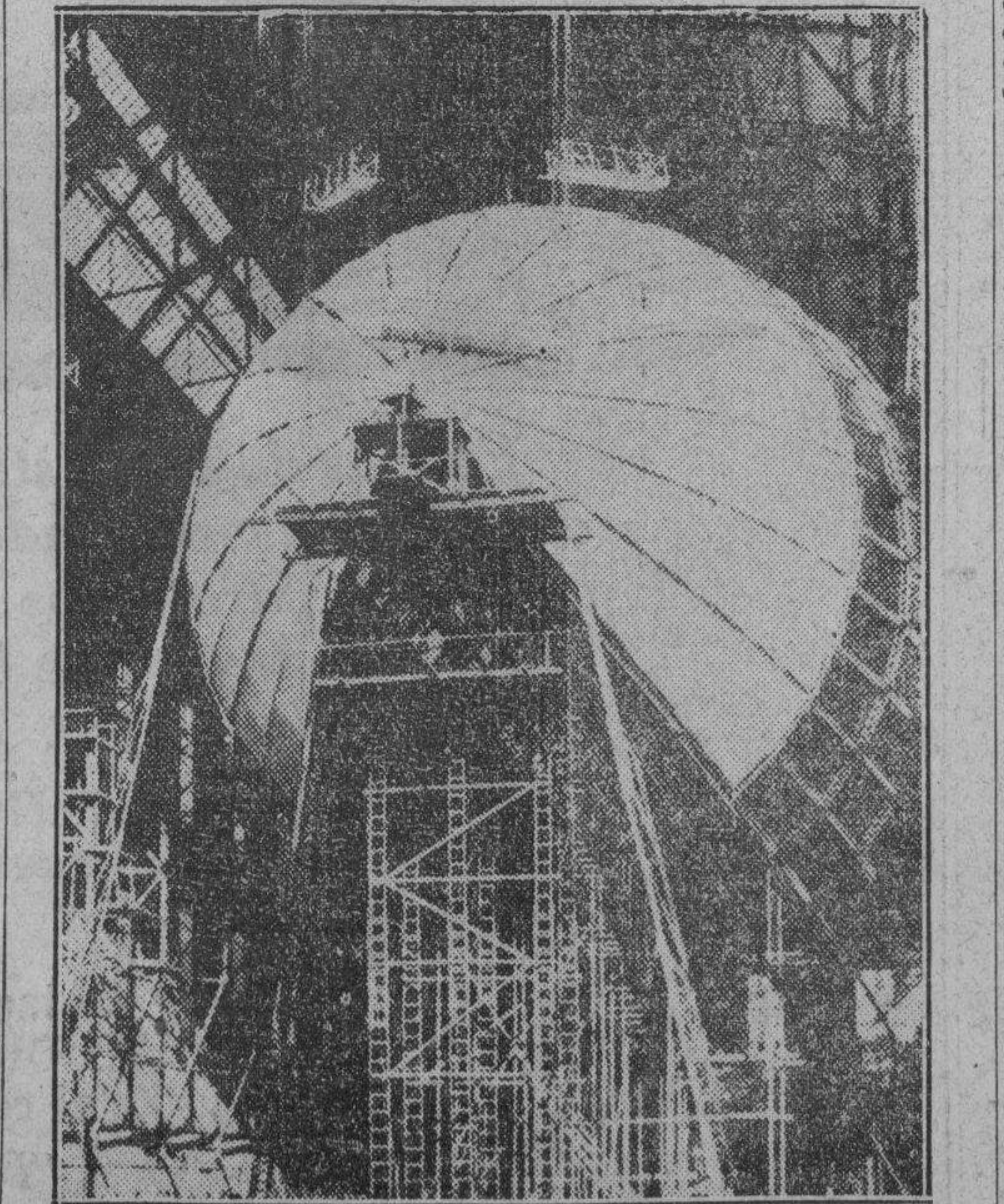
Un poco mas grande que el dirigible americano Macon, y dos veces mas grande que el Graf Zeppelin, este nuevo monstruo del aire, el LZ-129, esta por terminarse en Friedrichshafen, Alemania.
