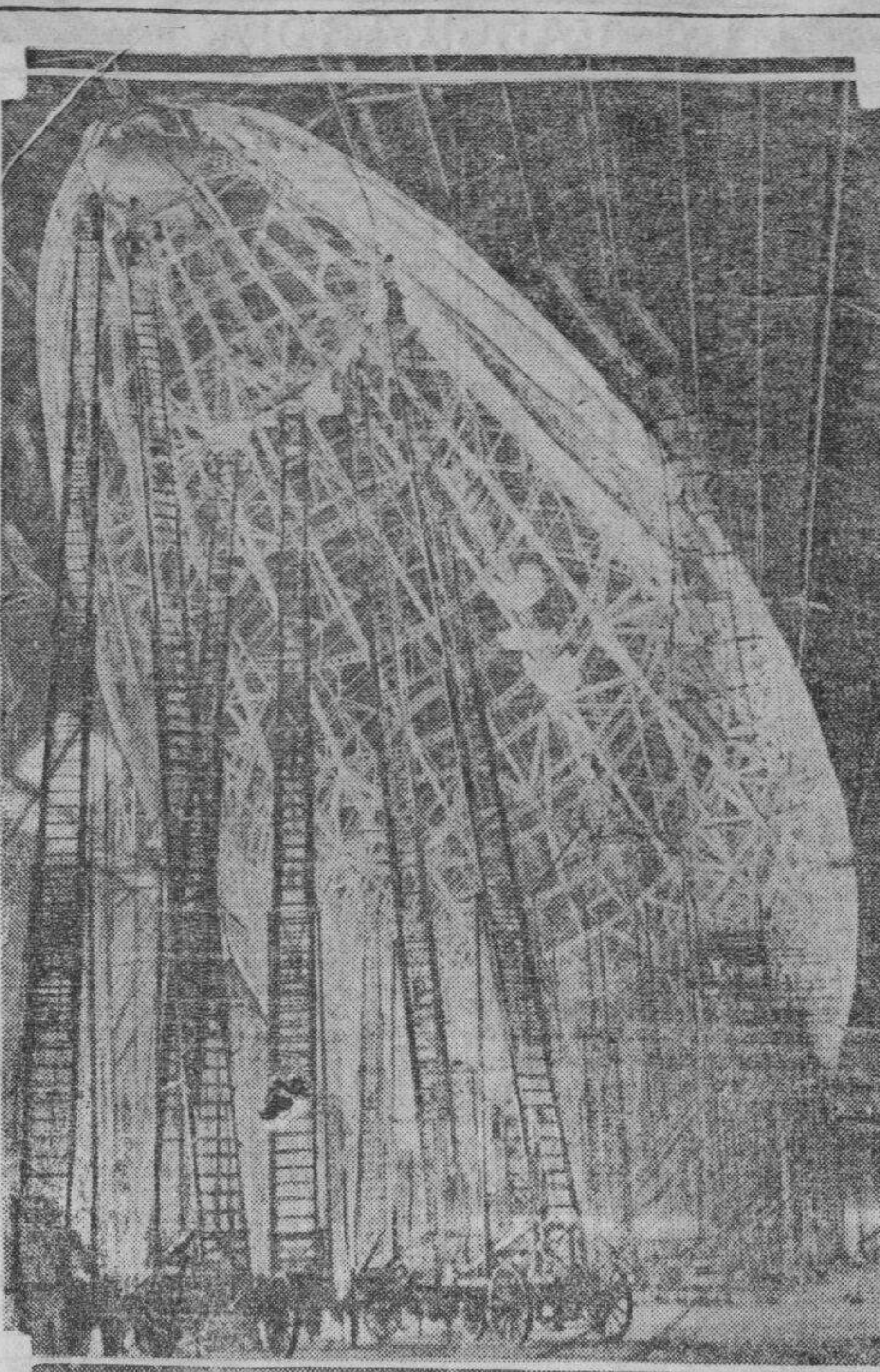
Obreros en actividad febril, en el hangar de Akron, Ohio, comenzando a instalar la cubierta exterior del gigantesco armazon del "U. S. S. Macon"...
