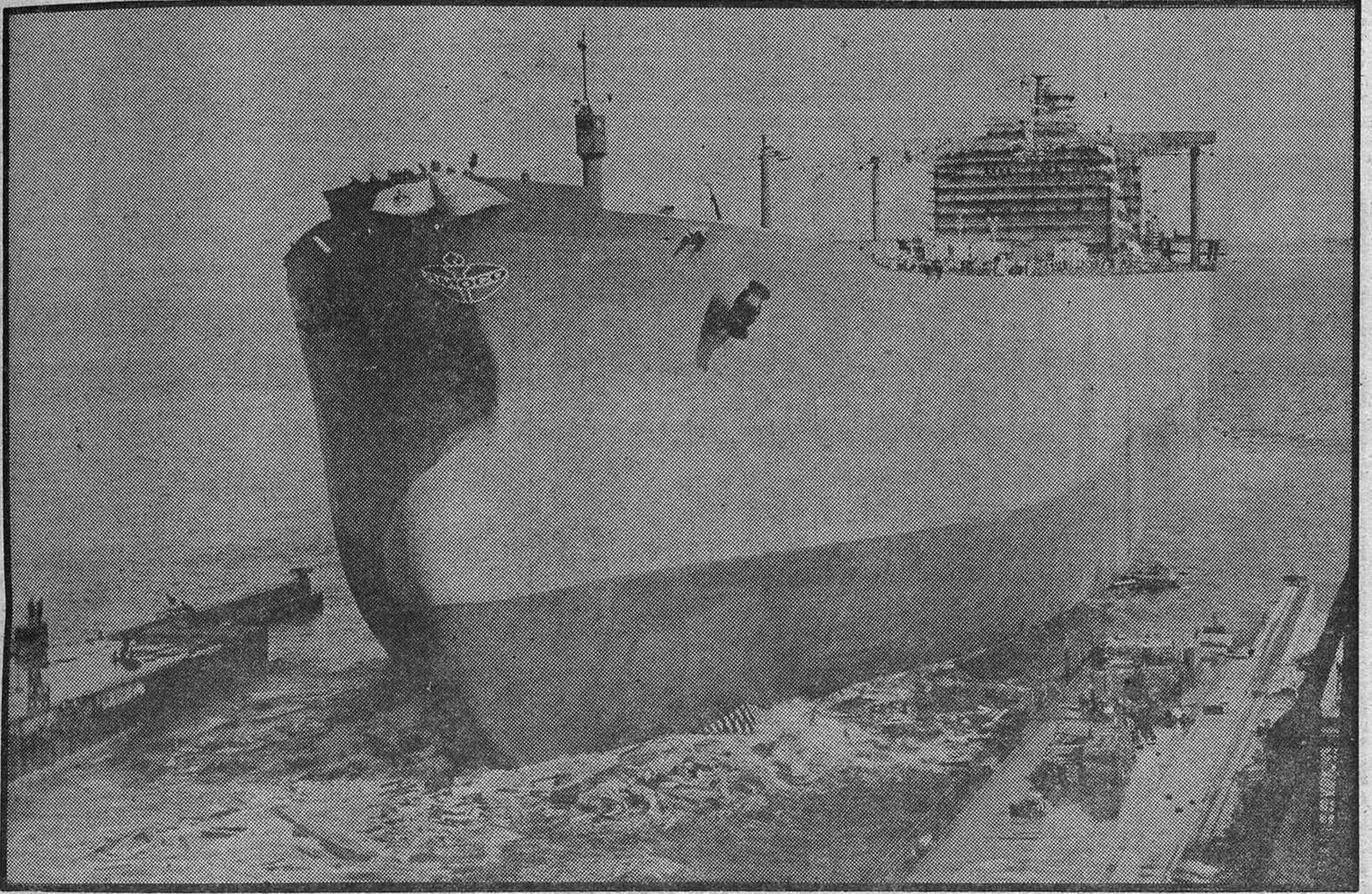
Uno de los gigantes de la "nueva generación" de transportes petrolíferos: el "Amoco Cádiz", de 230.000 toneladas de peso muerto, construido en la factoría de Cádiz de Astilleros Españoles
