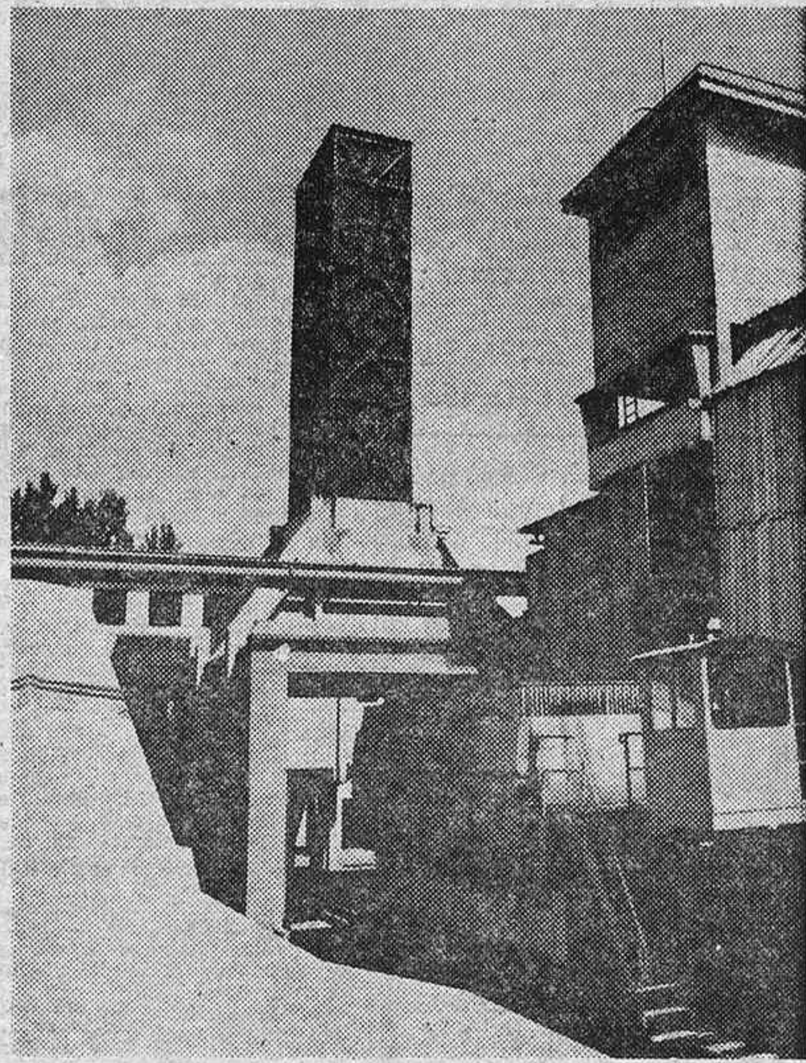
Carro de coque y torre de apagado en el Instituto del Carbón, en Oviedo
