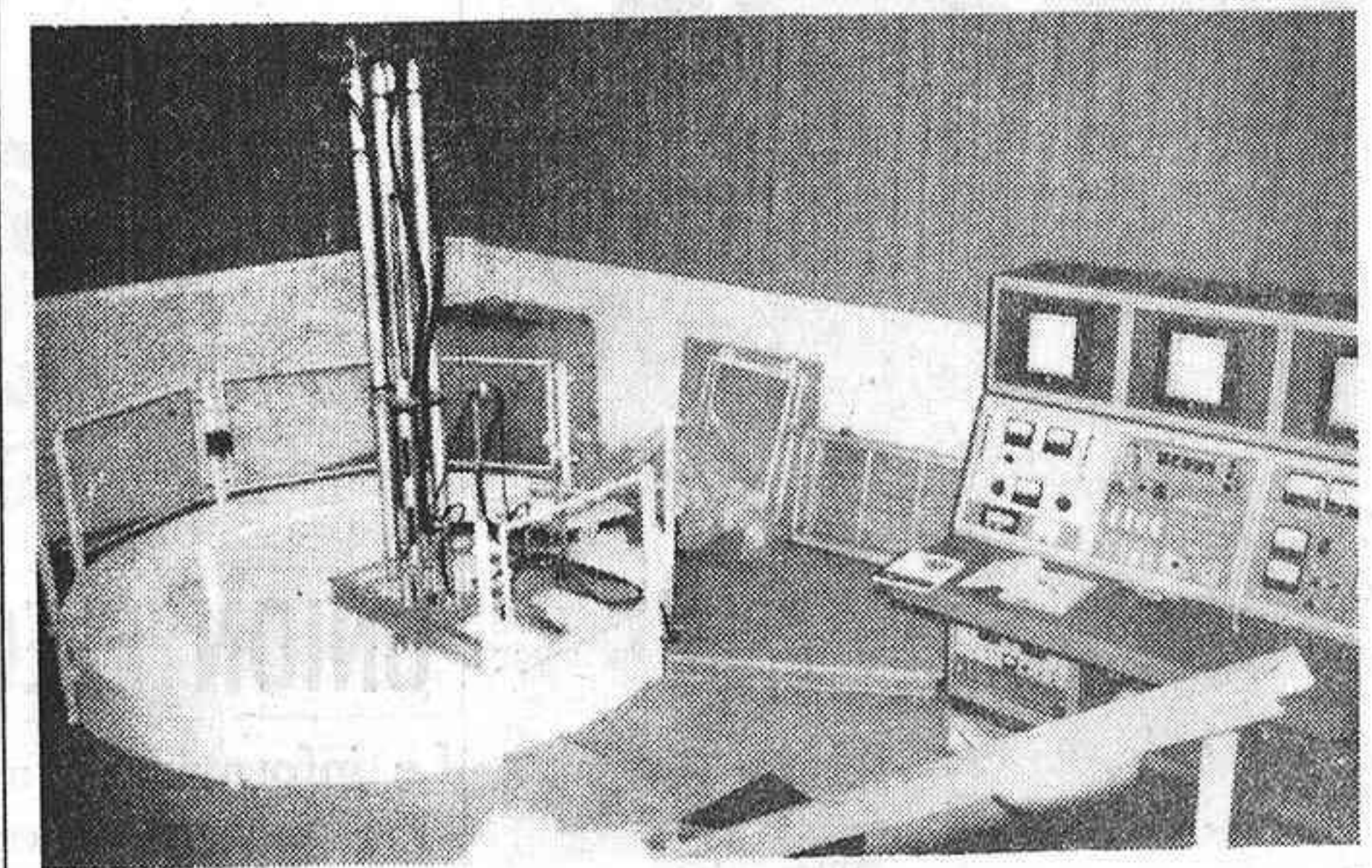
Reactor nuclear de diez kilovatios montado en la exposición Atomos en Acción, que se inaugurará el próximo día 16. (Foto Portillo.)
