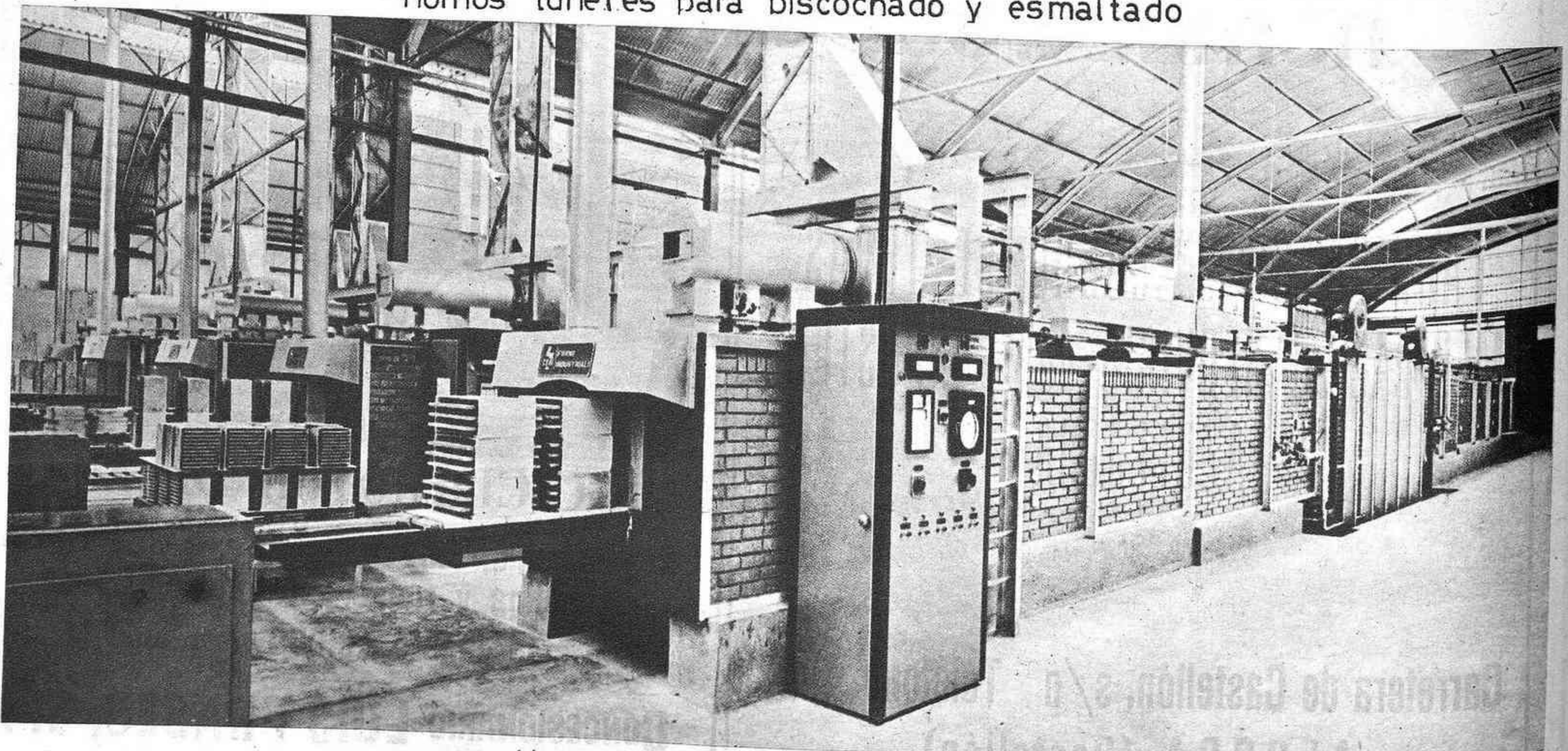
Hornos bicanales para esmaltados
