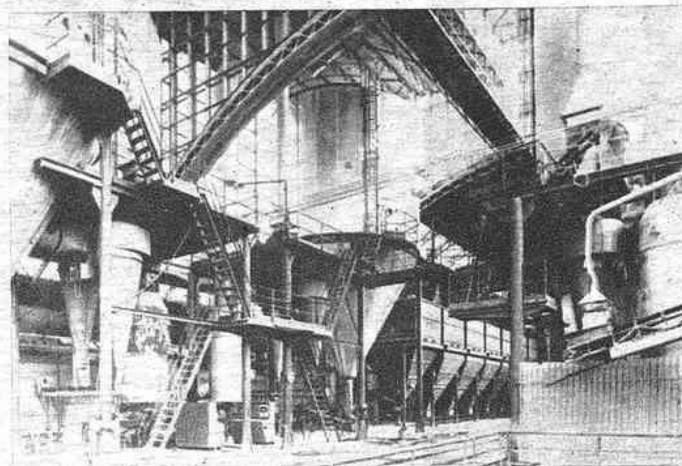
ATOMIZADOR
