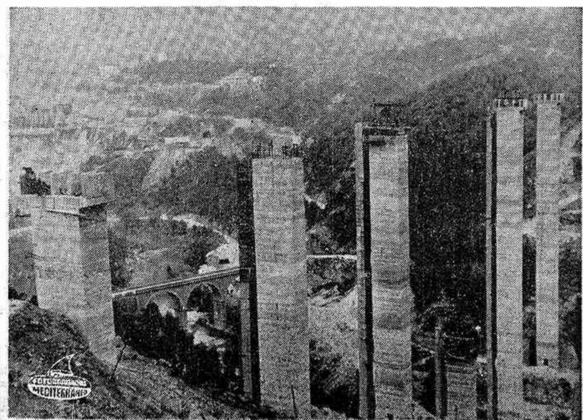
LA BAELLS (Barcelona). — Vista de los trabajos para la construcción del pantano de La Baells, en la comarca del Bergadán, y de un viaducto sobre dicho pantano, de 400 metros de longitud y una altura de 90 metros. — (Foto Cifra Gráfica).
