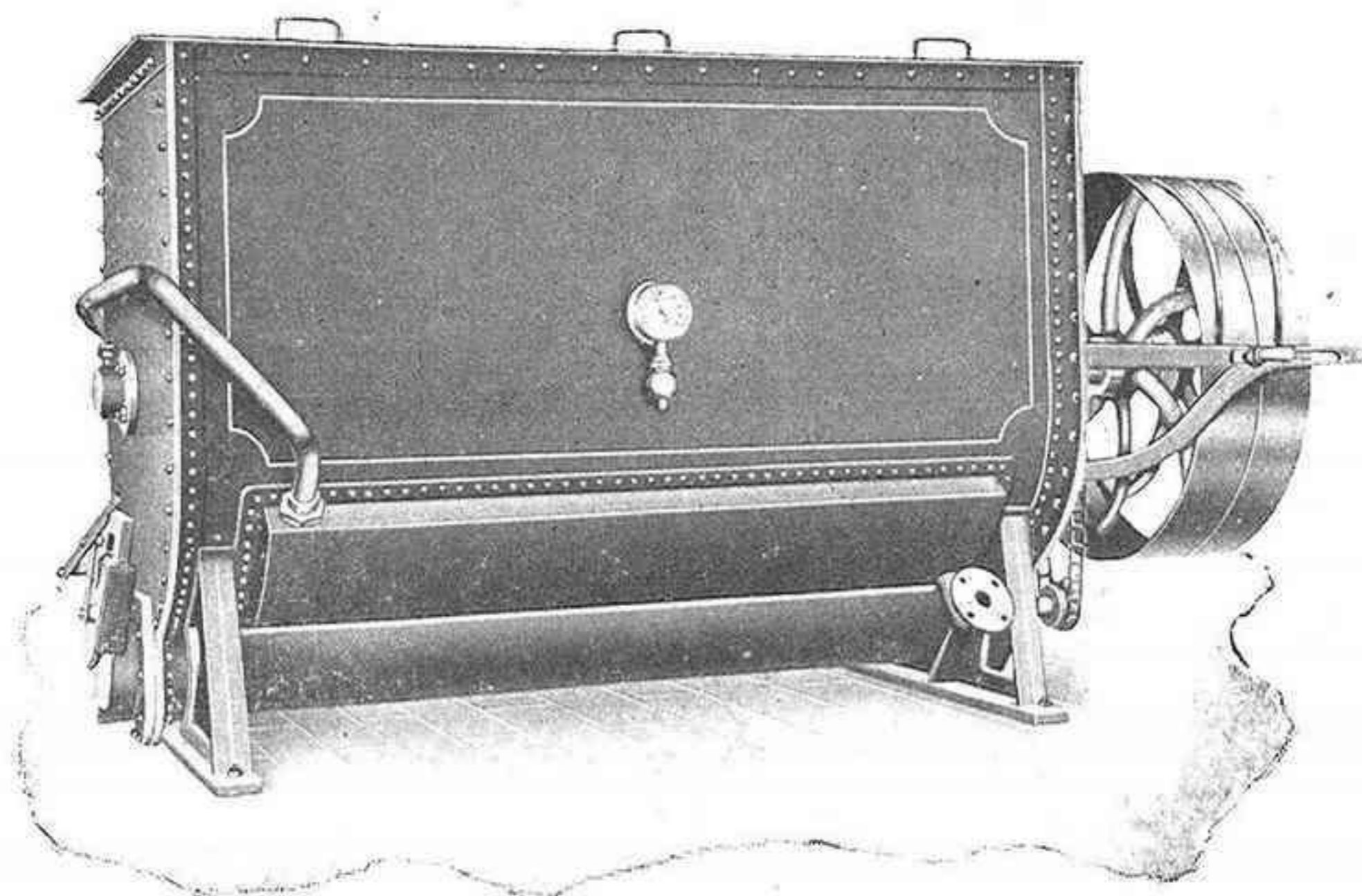
Termo-batidora para masas de aceituna
