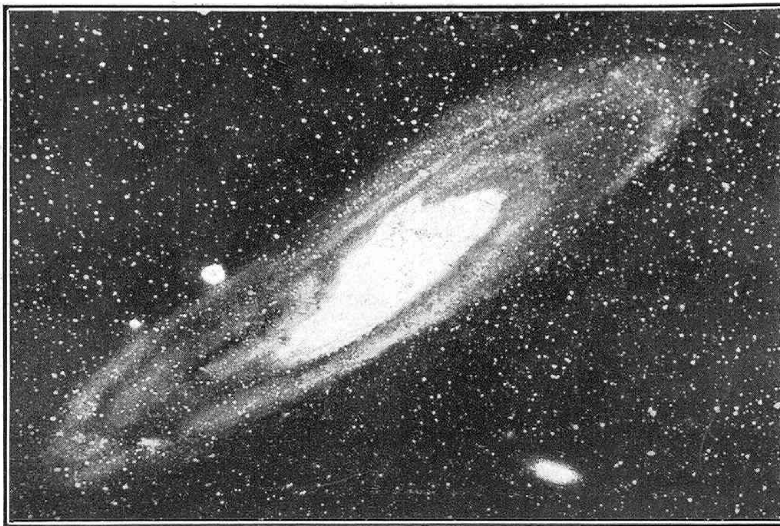
Núm. I.—Nebulosa elíptica de Andrómeda
