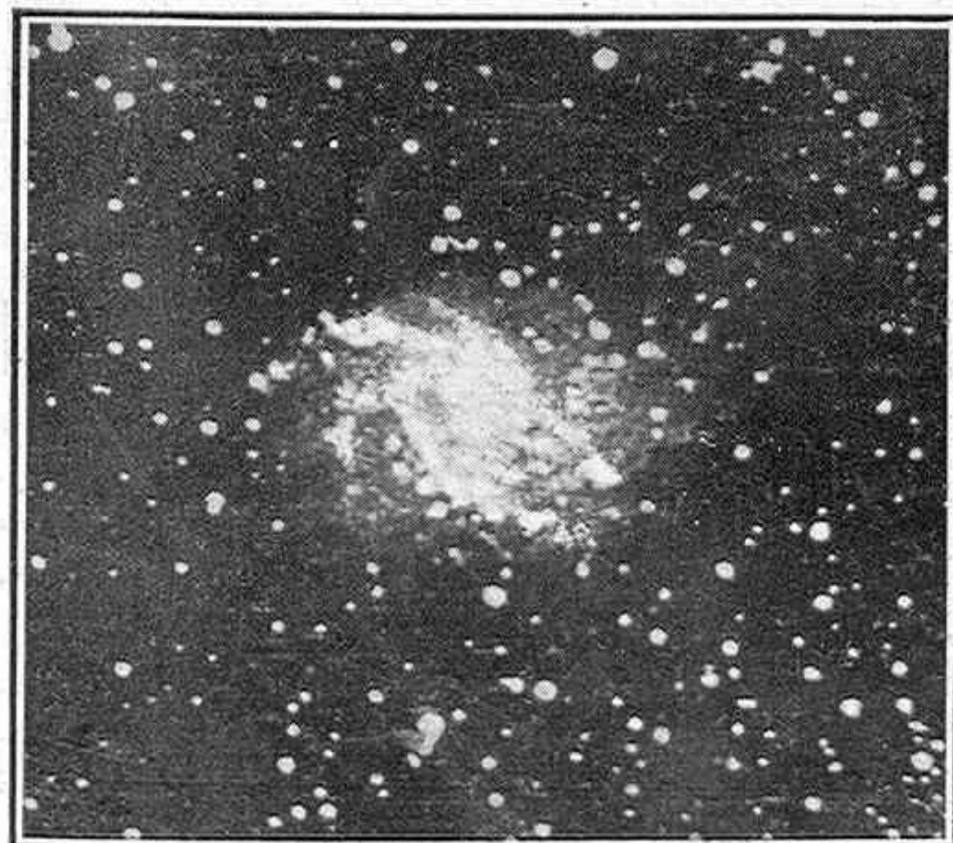
Núm. III.—Estérica de "Cefeo"
