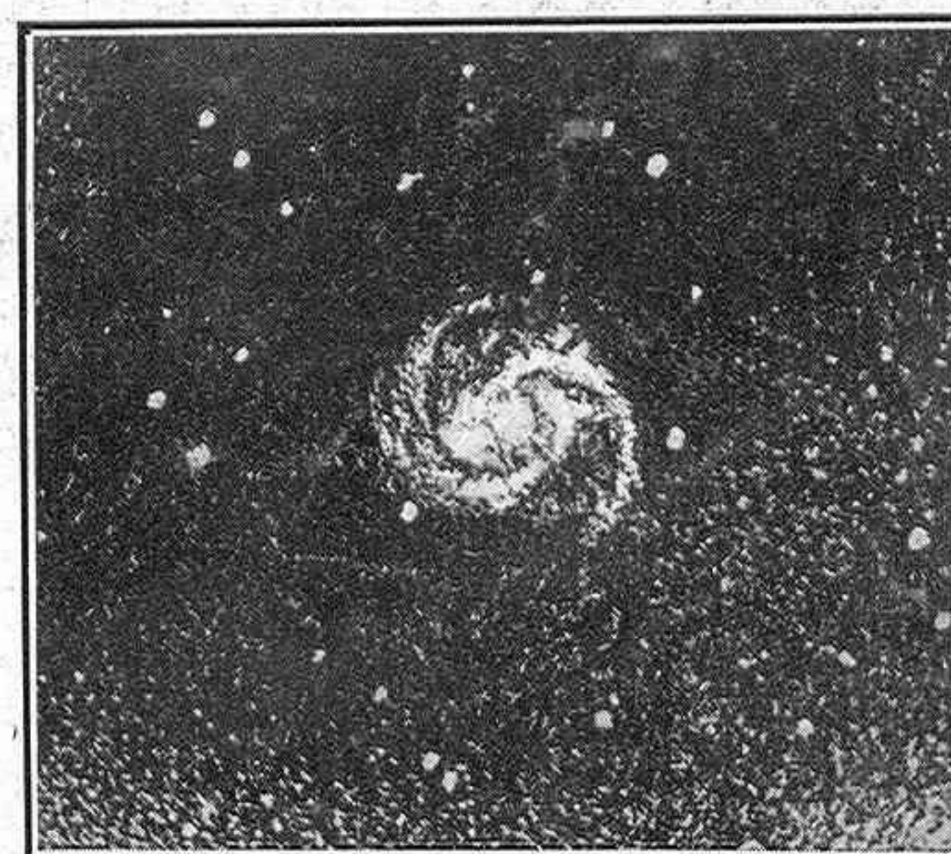
Núm. IV.—Torbellino en la "Constelación de Coma"
