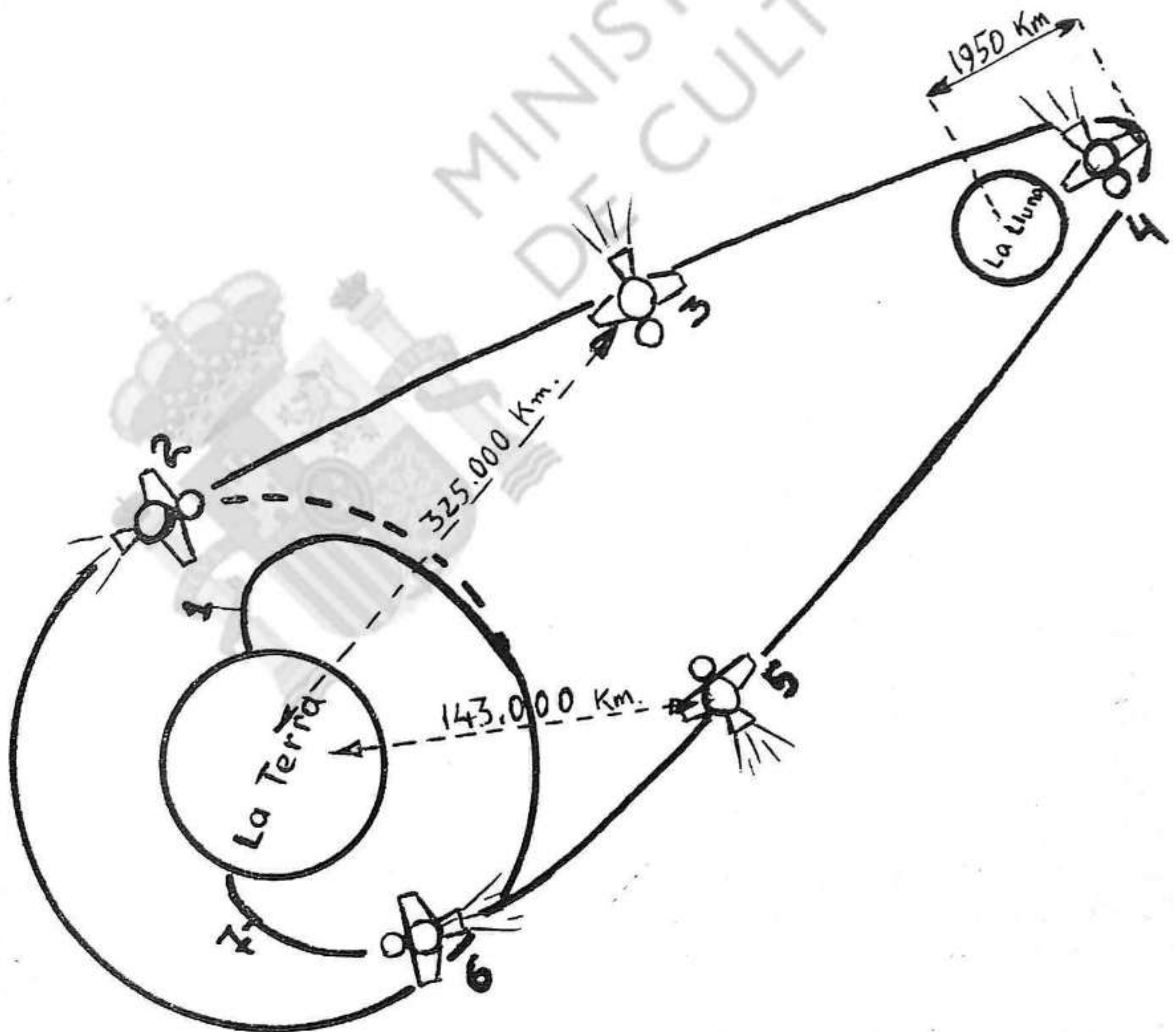
ESQUEMA DEL VOL DE L'ESTACIÓ AUTOMÀTICA «ZOND-5»: 1) Posta en òrbita intermitja. 2) Impuls cap a la Lluna. 3) Correcció de trajectòria. 4) Circumvol de la Lluna. 5) Segona correcció de trajectòria. 6) Separació del A.D. 7) Descens balístic a l'atmòsfera.
