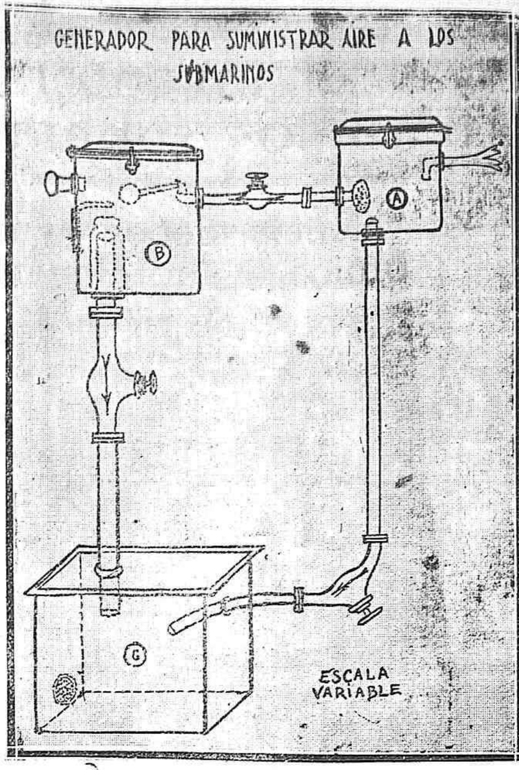
Esquema de los aparatos instalados en la cámara del tanque mediante los cuales verifica la extracción del oxígeno
