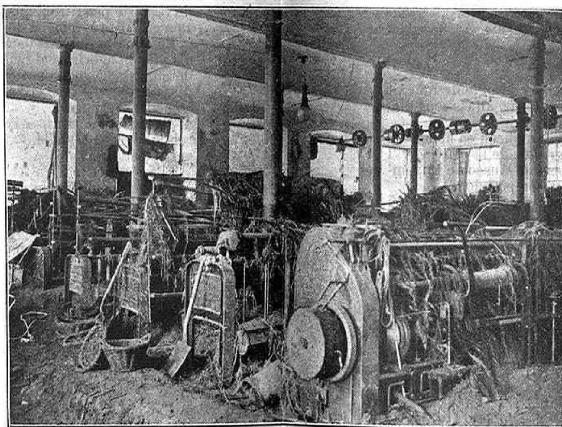
Com va quedar la sala de preparació de la fàbrica del Pont Vell.
