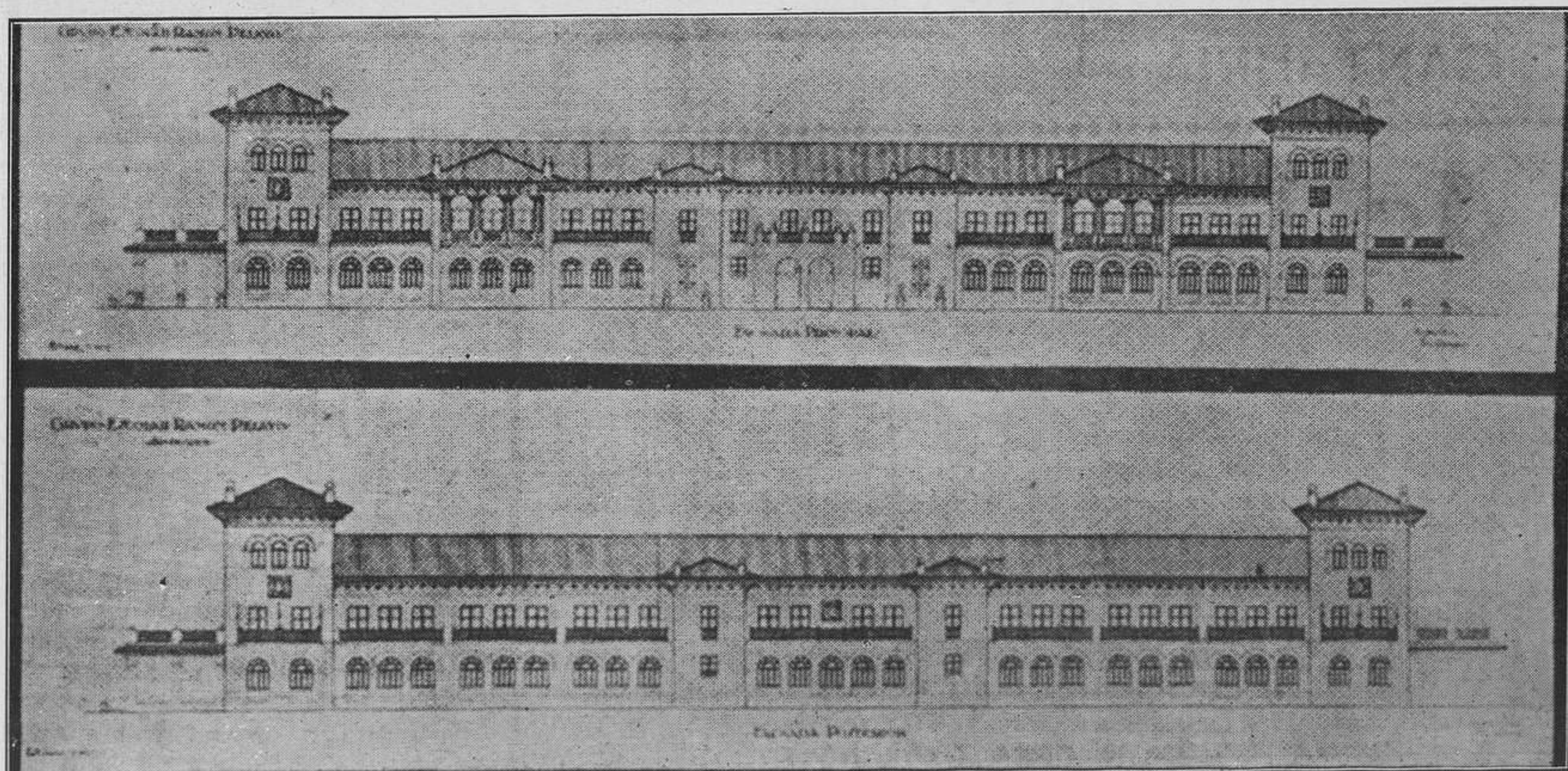
Proyecto del Grupo Escolar "Ramón Pelayo" que se está construyendo en Santander. Fachadas anterior y posterior.
