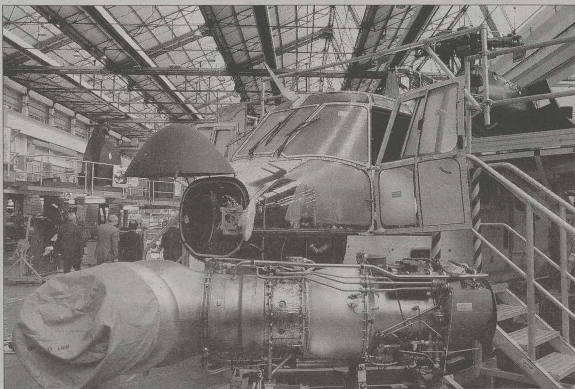
Una turbina de helicóptero, a punto de ser instalada en un aparato en construcción. / EUROCOPTER
