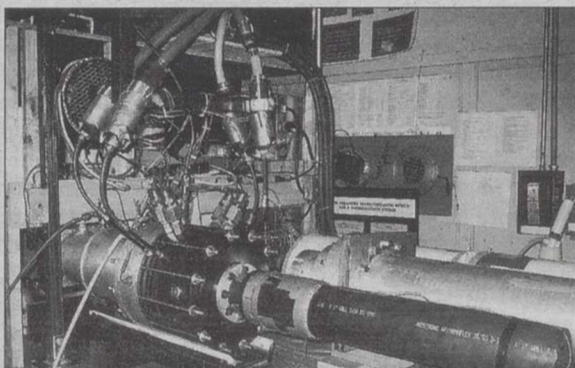
Prototipo de refrigerador termoacústico, universidad estadounidense de Purdue, Indiana, USA.
