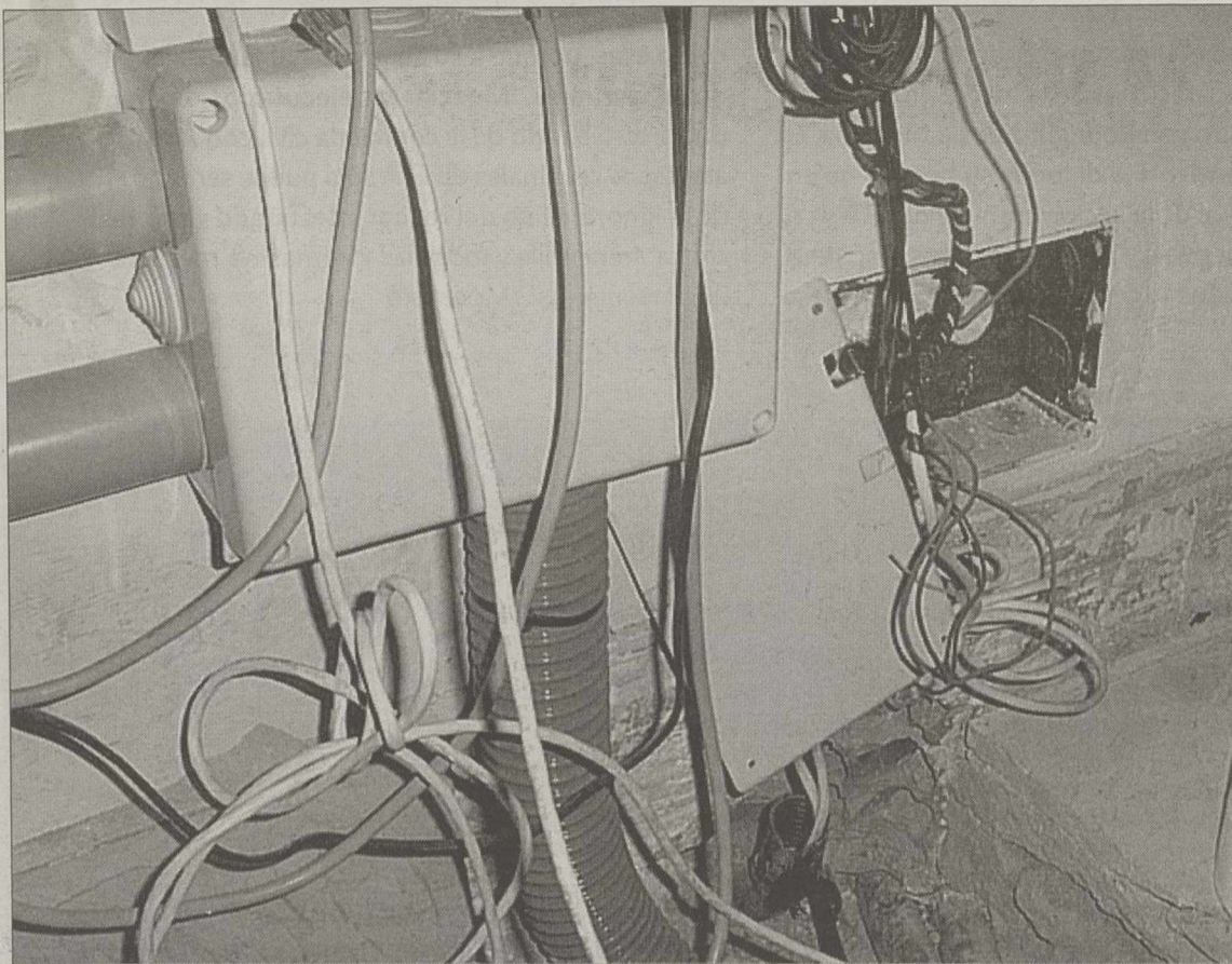
Entre las carencias detectadas figura la existencia de cuadros eléctricos con falta de señalización y rotulación. / LA TRIBUNA
