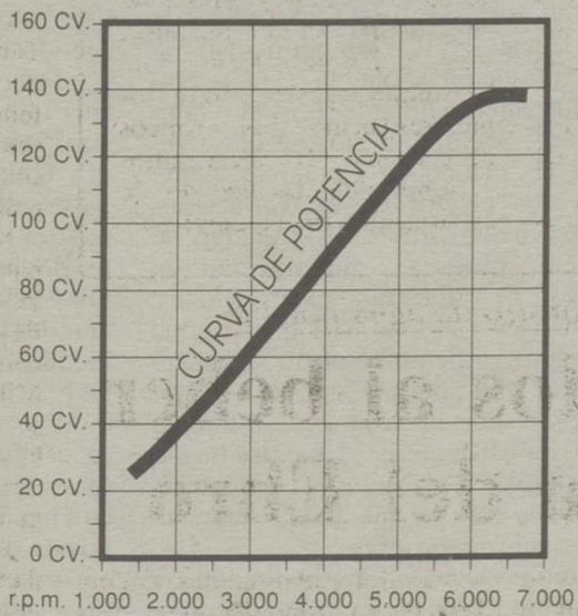
Potencia máxima obtenida: 140 CV a 6.500 r.p.m. La gran verticalidad de esta curva, expresa la facilidad de acceso a la zona de elevadas potencias, a un régimen motor razonable, alcanzando un máximo de 140 CV.
