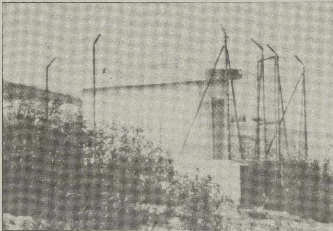
Estación sísmica automática ubicada en la localidad de Vianos, Albacete.
