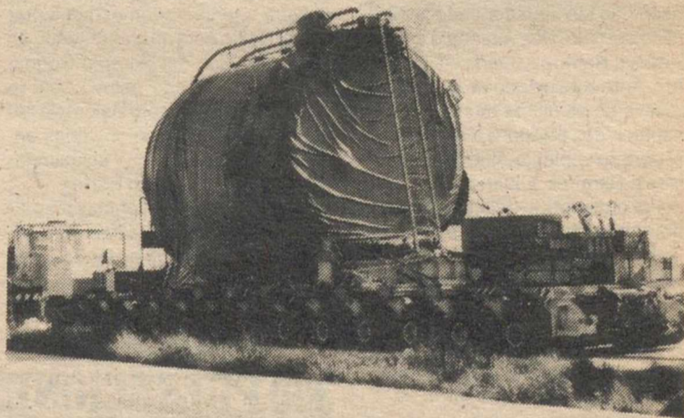
La vasija de presión del reactor sobre la gran plataforma de más de cincuenta metros de longitud.
