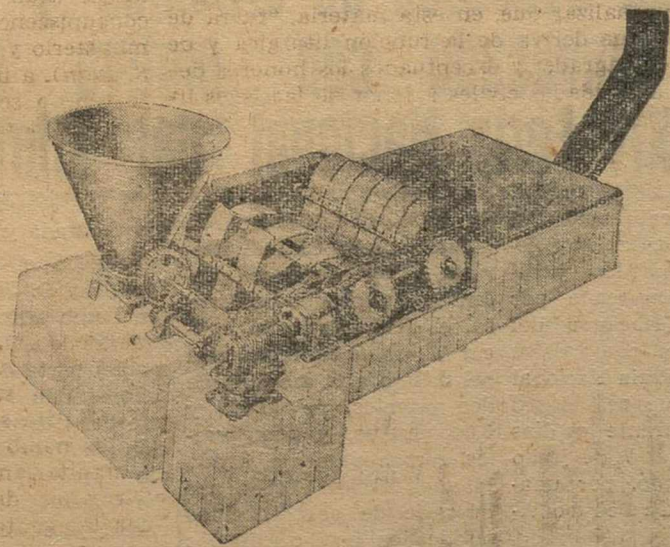
LAVADORA DE ACEITUNAS
