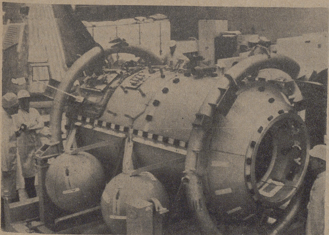
DOWNEY (California).—Este es el módulo de ensamblaje que conectará las aeronaves soviética y norteamericana durante el vuelo conjunto que el Apolo y el Soyuz realizarán en el año 1975.—(Telefoto AP EUROPA PRESS).
