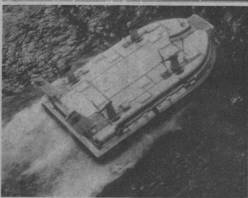
Dover.—El «SRN-4», de la clase «Mountbatten», el mayor aerodeslizador del mundo, sobre las aguas del canal de la Mancha, durante su viaje inaugural entre Dover y Bolegnes. El «SRN-4» alcanza velocidades de hasta 96 kilómetros por hora y puede transportar doscientos cincuenta pasajeros y treinta automóviles.—(Telefoto AP-Europa Press)
