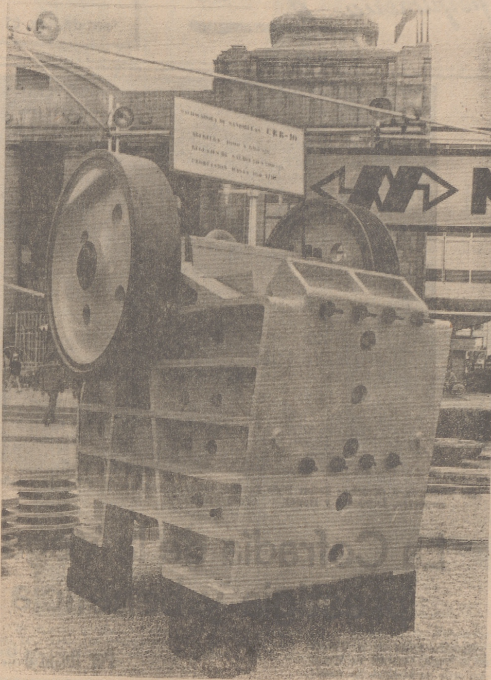
He aquí una extraña máquina que se expone en la Feria Internacional de Muestras de Barcelona. El letrero colocado sobre ella dice: «Machacadora de mandíbulas». Reglajes de salida 80 a 200 m/m. Producción hasta 180 T/H. ¿Pero qué clase de mandíbulas son las que machaca...? (Foto fiel).
