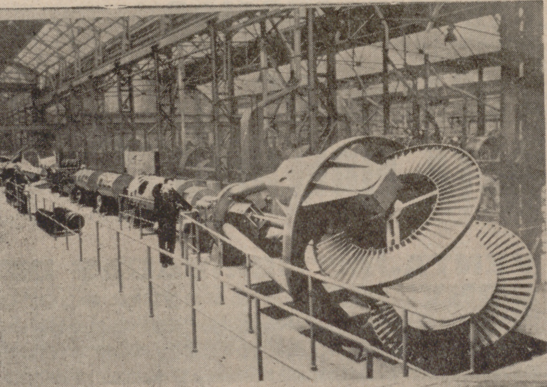
HAMBURGO. (DaD).—Las mayores máquinas de cables de alta tensión del mundo las recibirá el Japón de la República Federal de Alemania. La casa Krupp suministrará a las empresas japonesas Furukawa Electric y Showa Electric cableadoras de una longitud de 47 m. y de un peso de 63 toneladas, capaces de producir cables de alta tensión de hasta 127 m. de diámetro para la alimentación de corriente.
