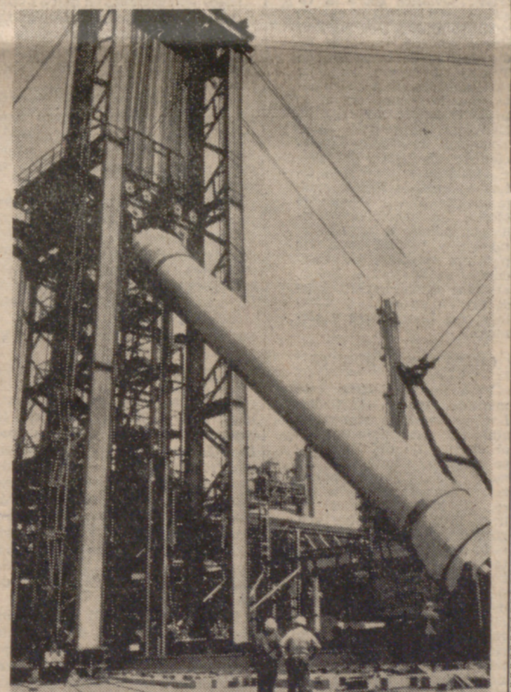
LUDWIGSHAFEN. (DaD).— Este reactor de 23 metros de altura es la pieza más grande del mundo para reactores de alta presión. El coloso tiene un diámetro de 2,50 metros y un peso de 400 toneladas. Fue construido, transportado e instalado por cuenta propia por una agrupación de empresas químicas en Ludwigschafen.
