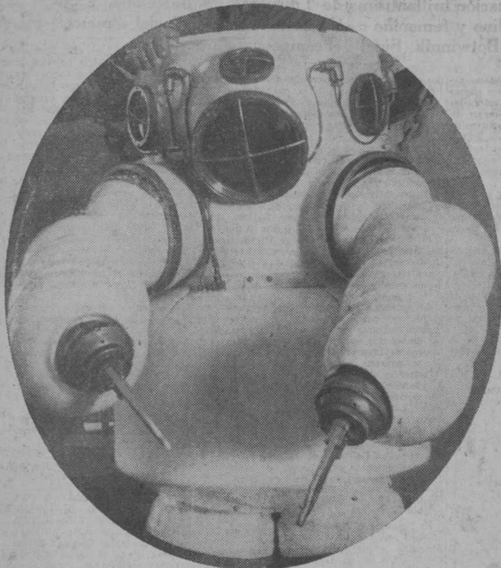
Un nuevo aparato para trabajos submarinos, construido por un alemán. Su coste aproximado es de 80.000 marcos y permite descender a una profundidad de 250 metros. Se utilizó con gran éxito en la búsqueda del cargamento de oro del "Egipto"
