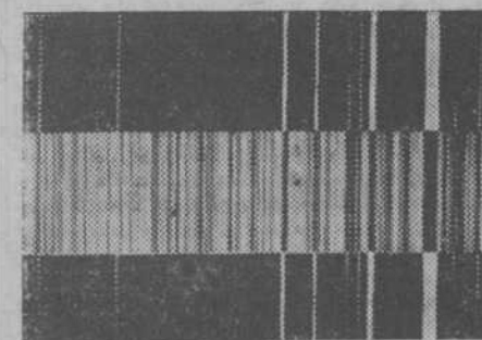
Identidad entre el compuesto químico, óxido de titanio, ensayado en el laboratorio, y este mismo cuerpo en la estrella Betelgeuse, a una distancia que raya en los tres mil billones de kilómetros
