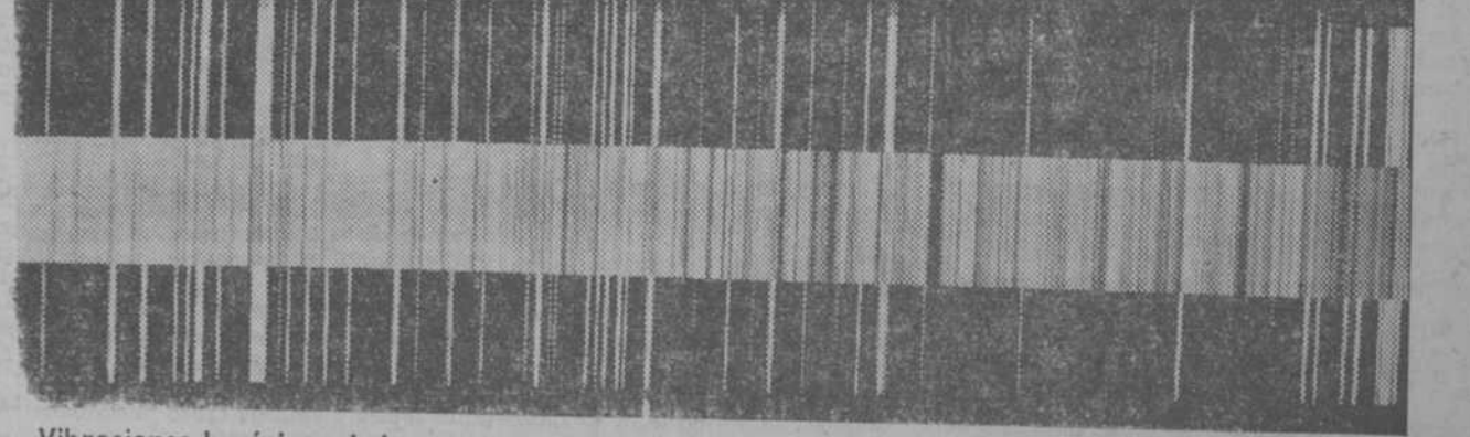
Vibraciones luminosas de la estrella Aldebarán, que anduvieron durante sesenta años a la velocidad de 300.000 kilómetros por segundo, antes de impresionar la placa, junto con otros elementos químicos ensayados en el laboratorio
