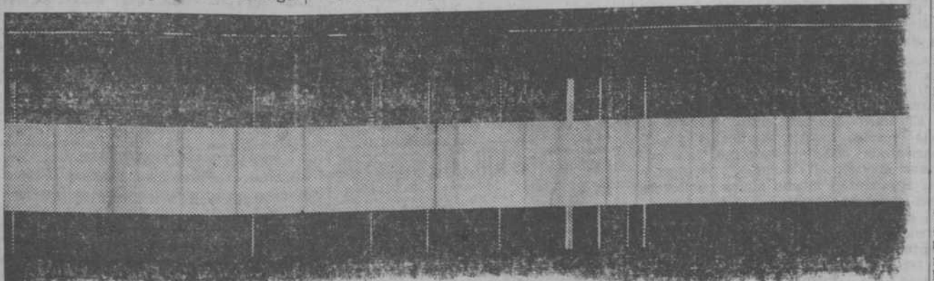
La estrella Epsilon en la constelación de los Lebes, con las rayas características del gas helio, el mismo que llena nuestros grandes dirigibles
