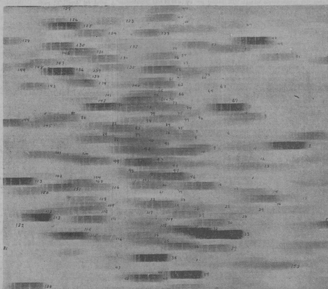
Abundancia de hidrógeno en el Cosmos; las rayas características de este gas aparecen en la mayoría de los soles proyectados en la constelación del Navio. Eddington estima que el hidrógeno integra por lo menos una tercera parte del peso total de las estrellas
