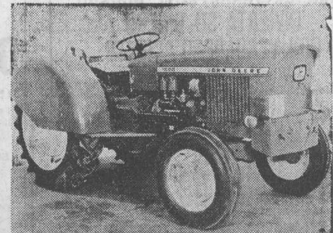
Nuevo tractor John Deere, modelo «1.020-LU-Compacto», de 47 CV, al motor, especialmente diseñado para la mecanización de nuestros viñedos y frutales.
