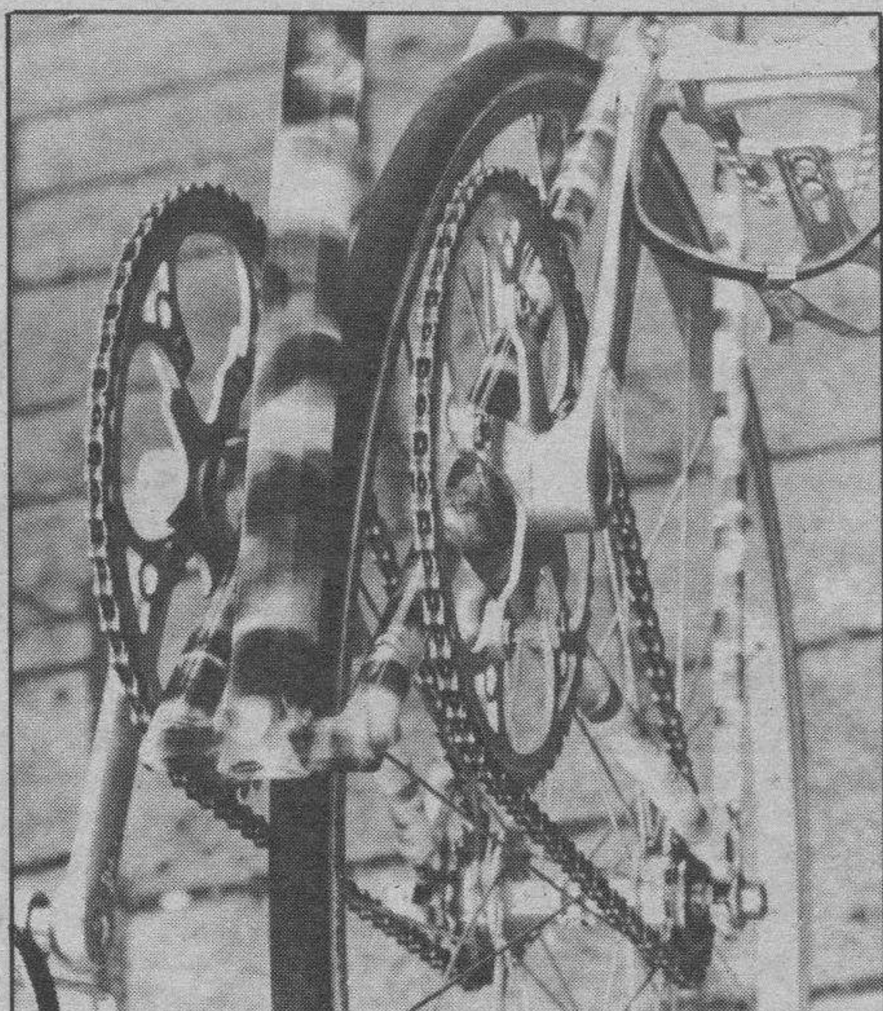
Aspecto detallado de las dos estrellas. La rueda trasera pasa por la caja pedalier.
