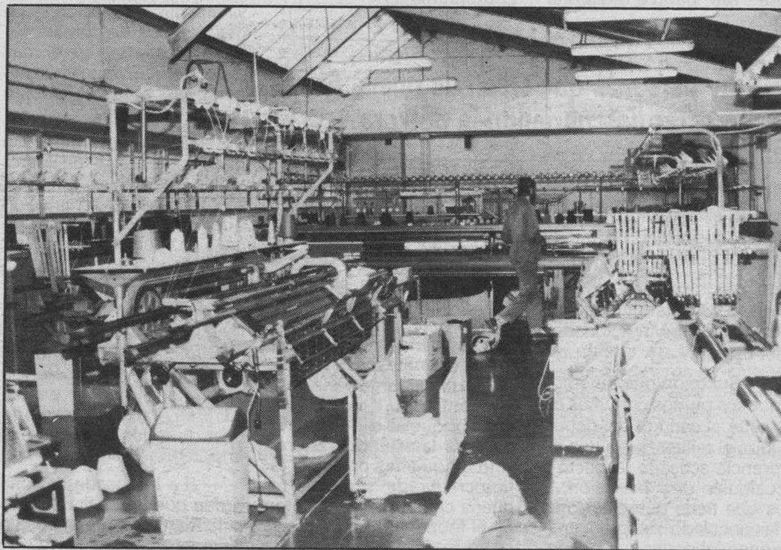
Vista de la fábrica e interior del taller.
