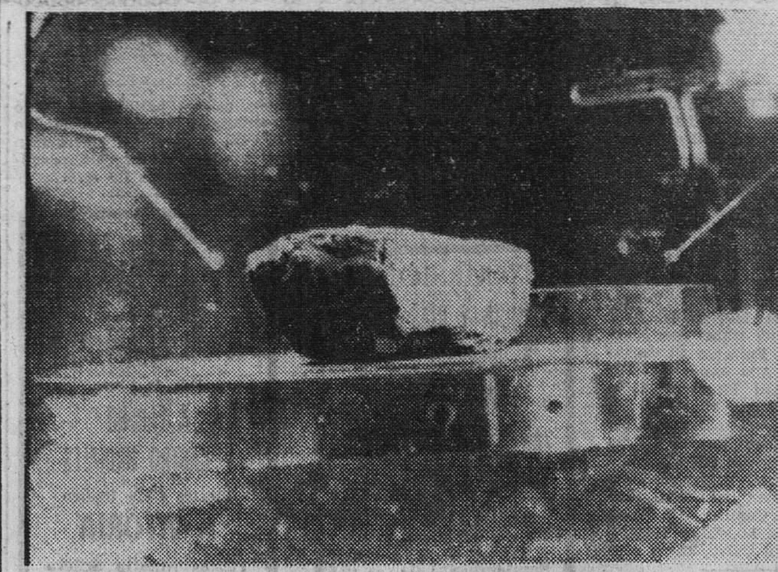
Centro Espacial de Houston (Tejas). — La NASA ha hecho pública esta fotografía que muestra una roca lunar, traída por los astronautas del «Apolo XI». Es ignea y los geólogos dicen que es similar en apariencia a muchas de la Tierra. Esta es la primera vez que la NASA hace público un primer plano de material lunar. (Telefoto UPI-CIFRA)
